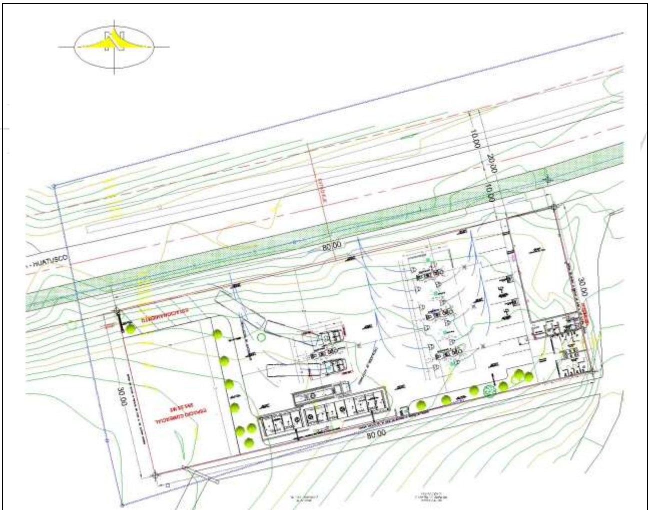
Figura 2. Plano de conjunto de la estación de servicio, a la altura del km 53+960 de la carretera Córdoba-Cardel, Tramo Fortín-Conejos en el Municipio de Totutla, Ver.
