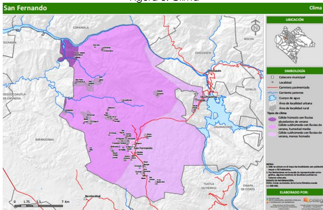
Figura 8. Clima
