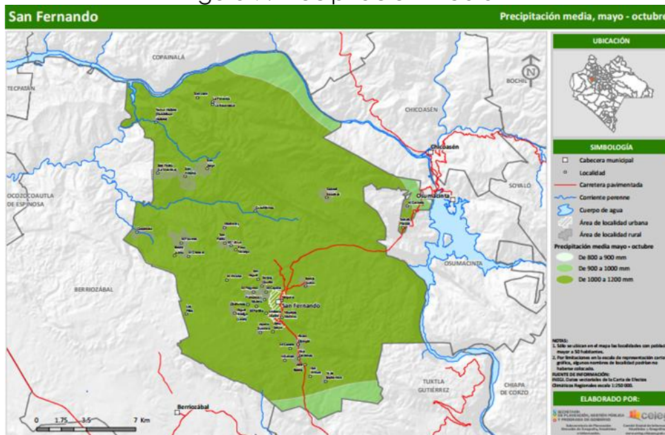
Figura 7. Precipitación media
