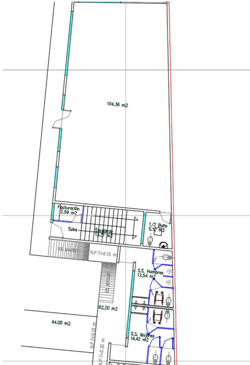
Ilustración 1. Extractos del Plano Arquitectónico del Proyecto
