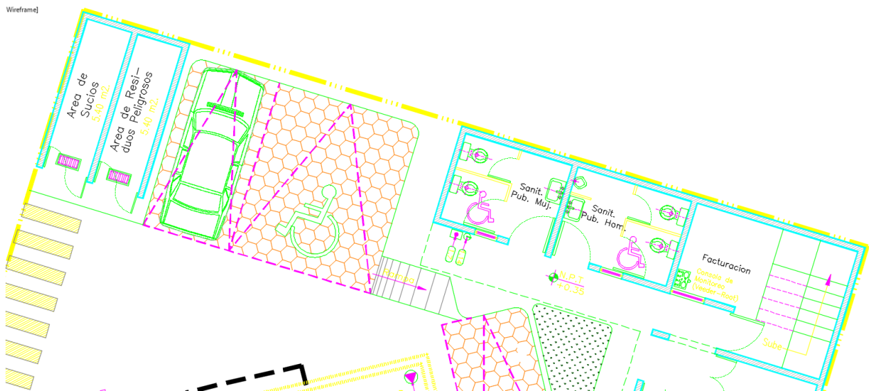
Ilustración 1. Extractos del Plano Arquitectónico del Proyecto
