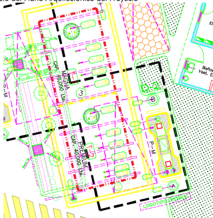
Ilustración 3. Extracto del Plano Arquitectónico del Proyecto
