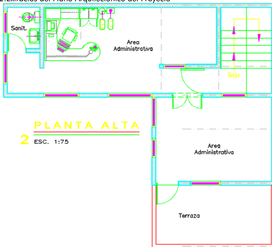
Ilustración 2.Extractos del Plano Arquitectónico del Proyecto
