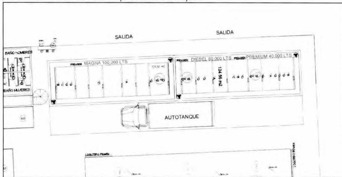
Ilustración 3. Extracto del Plano Arquitectónico del Proyecto
