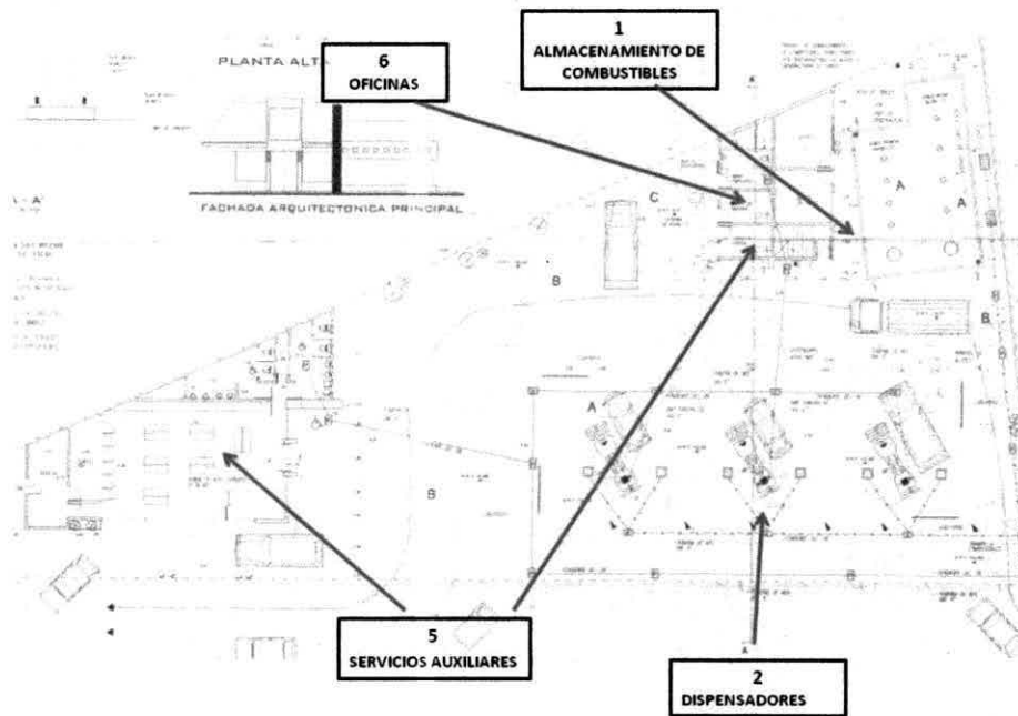
Diagrama 1 Diagrama de plano
