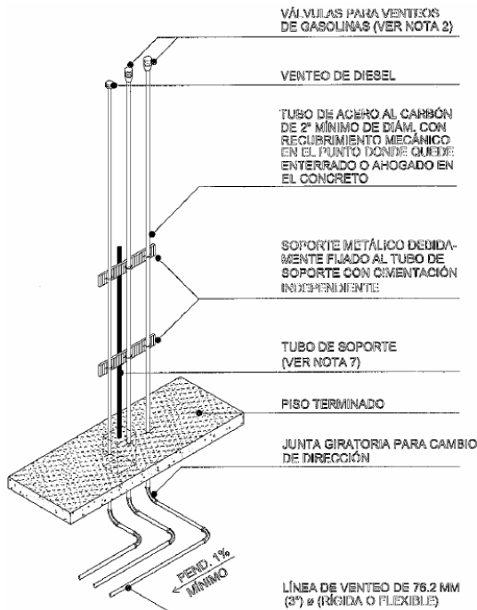
DETALLE DE VENTOS CON SOPORTE METÁLICO INDEPENDIENTE
