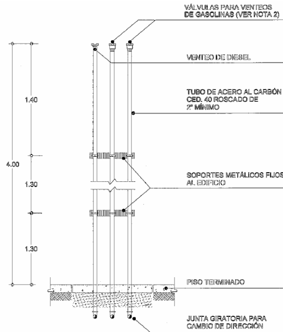
DETALLE DE VENTEOS ADOADOS AL EDIFICIO
