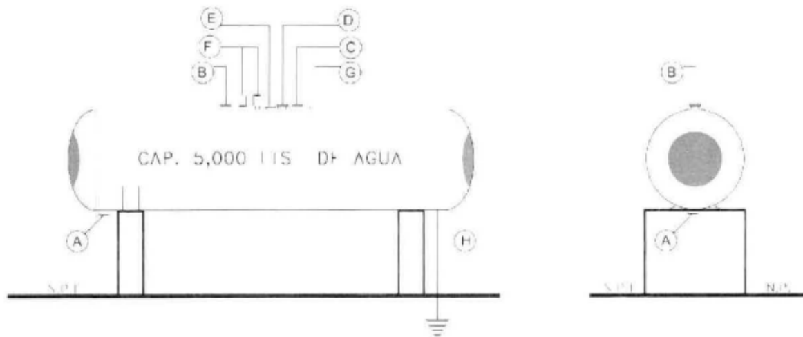
Figura 12. Instrumental de seguridad del tanque de almacenamiento.
