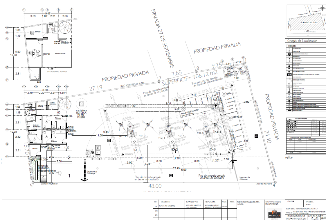
Imagen 12. Plano de Conjunto de ESTACION DE SERVICIO, "ENERGETICOS CIHUALPILLI S.A. DE C.V."
