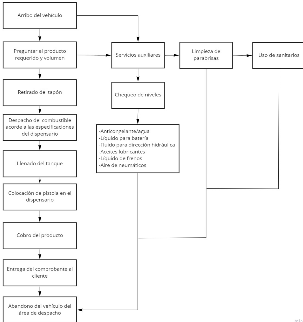
Diagrama 2: procesos para despacho de combustibles
