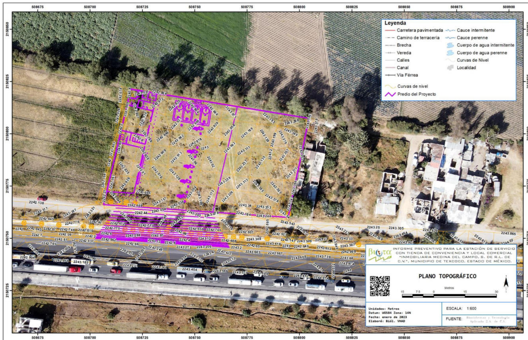
Imagen III. 34. Plano Topográfico para el Proyecto.
