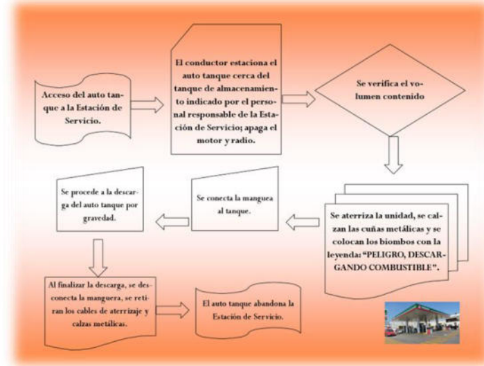
Imagen III. 5. Diagrama del proceso y procedimiento de operación.
