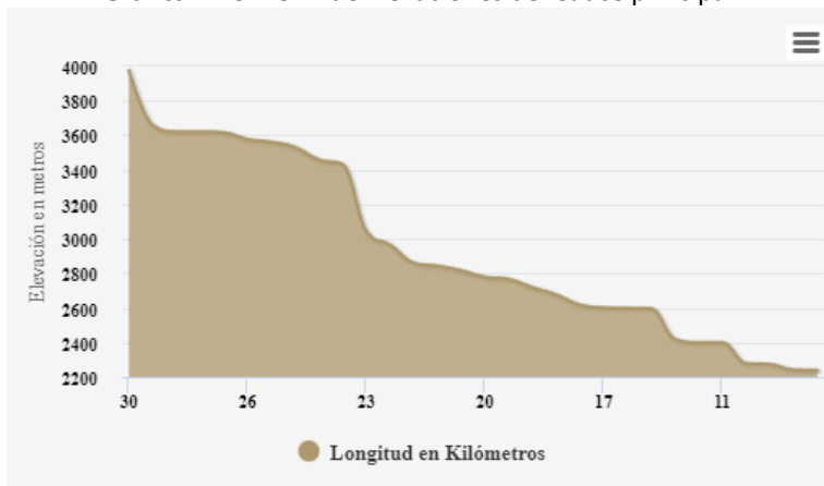
Gráfica III. 3. Perfil de Elevaciones del Cauce principal.
