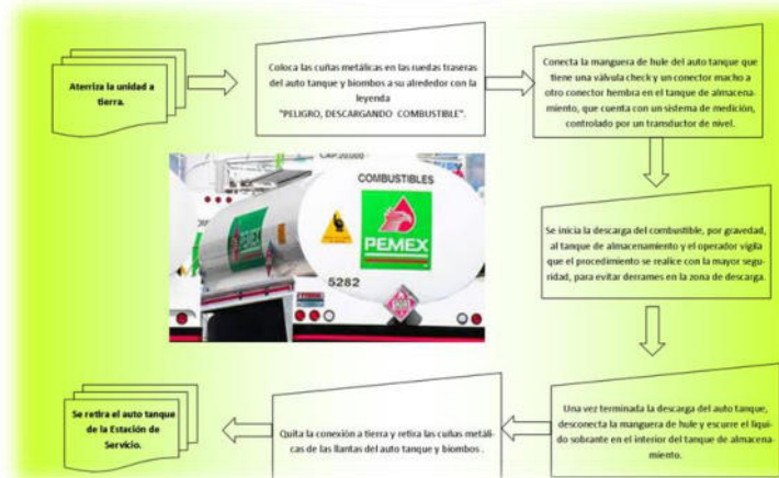
Imagen III. 6. Procedimiento de descarga en tanque de almacenamiento.
