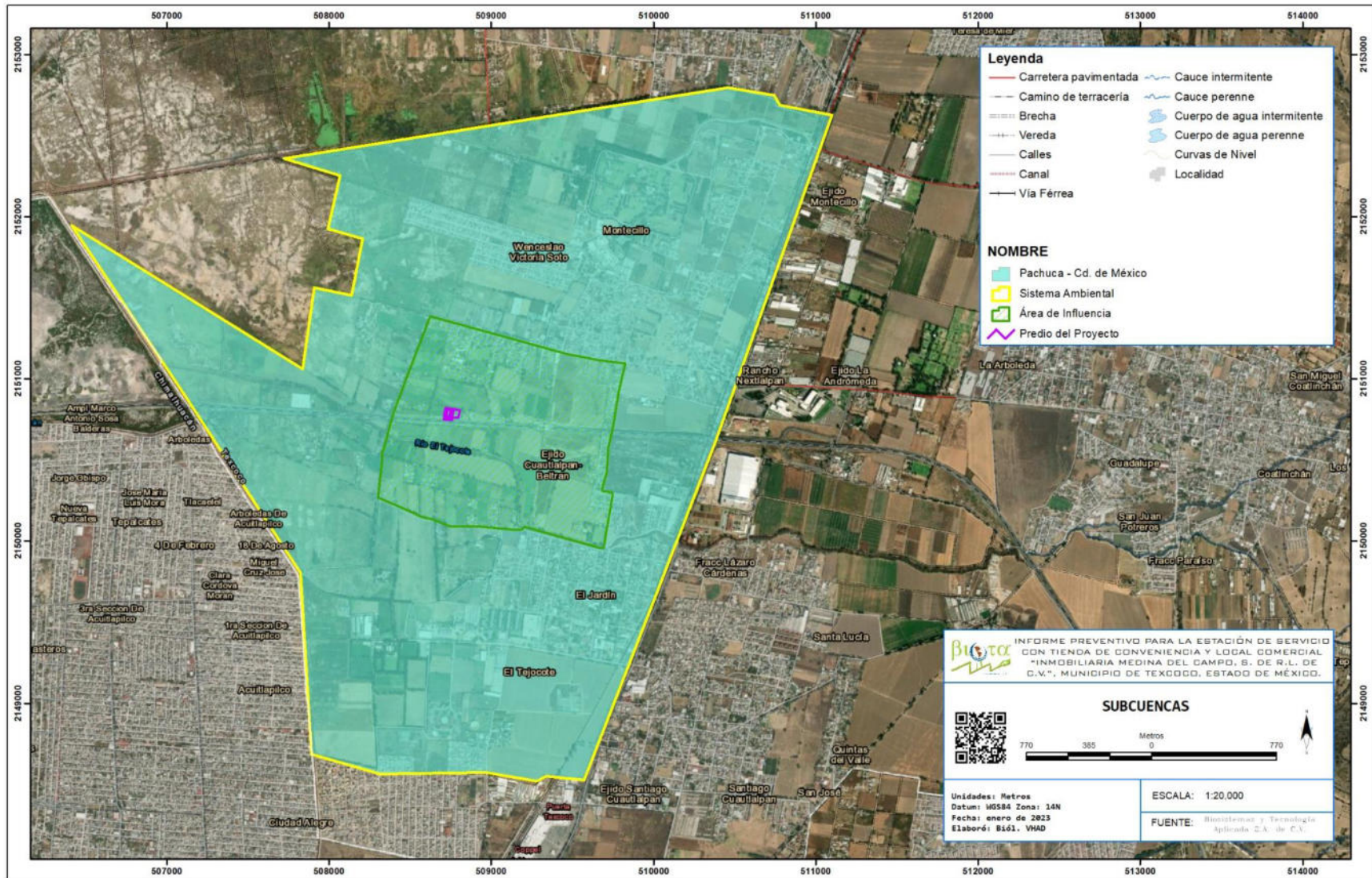
Imagen III. 41. Subcuencas Hidrológicas del Sistema Ambiental y Área de Influencia del Proyecto.
