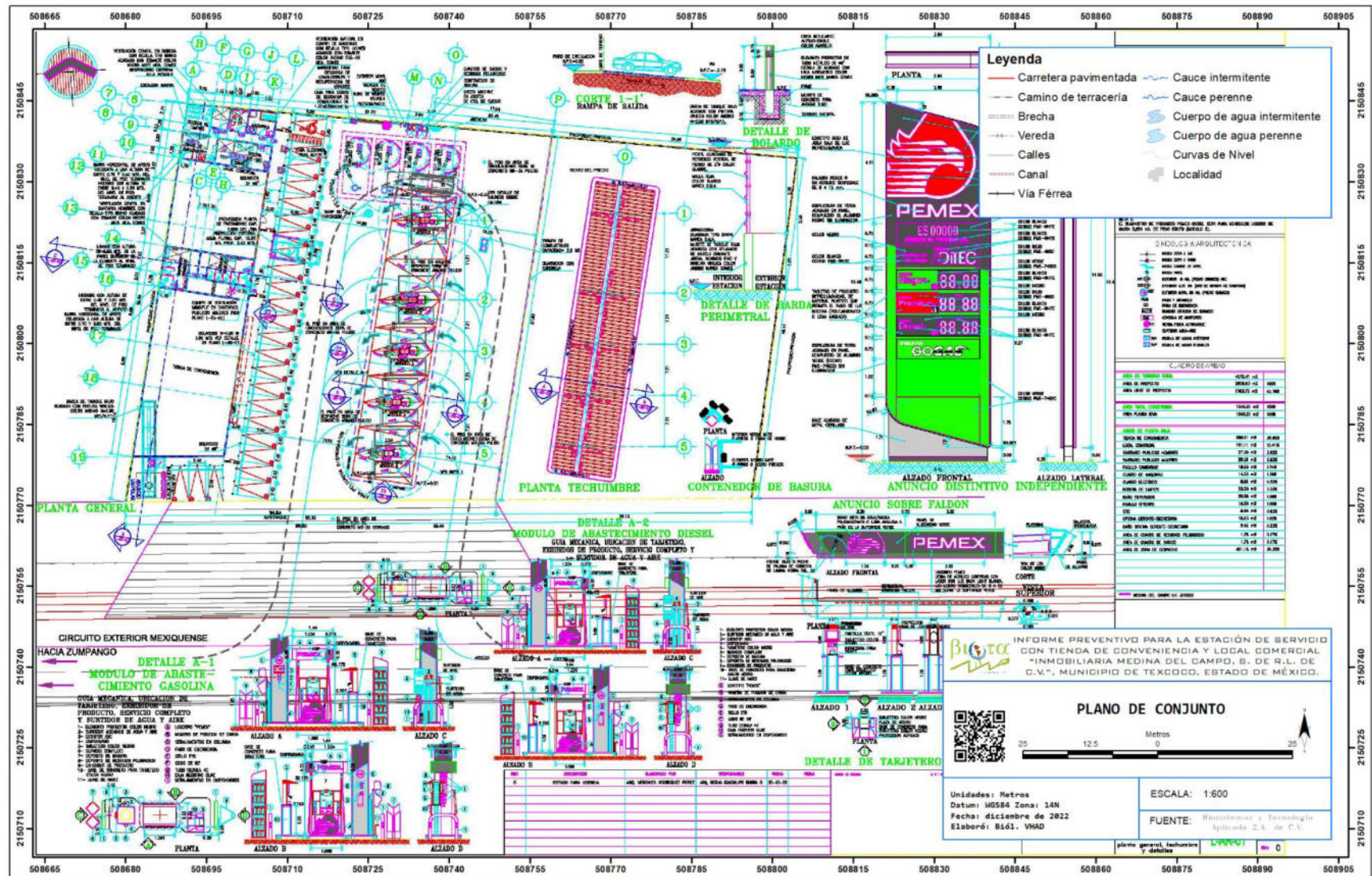
Imagen III. 2. Plano de Conjunto.
