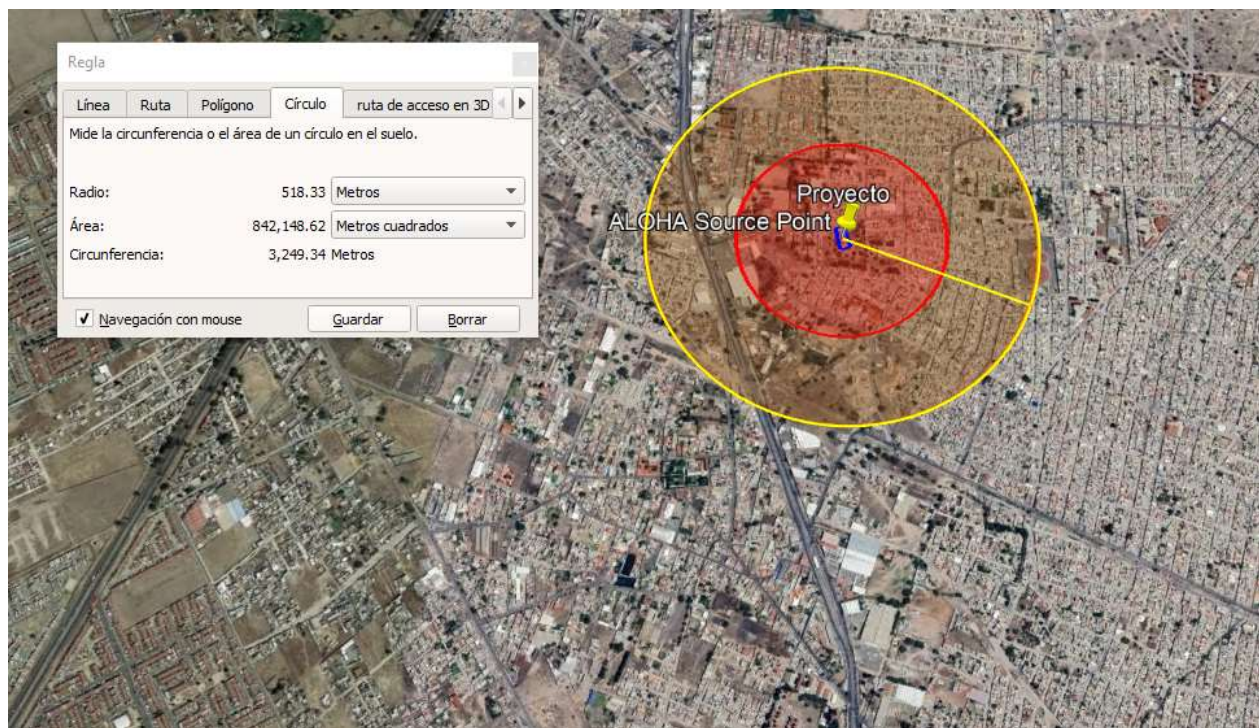
IMAGEN 11. Superficie de incidencia y afectación por escenario de Explosión de Vapores en Expansión de Líquido en Ebullición “BLEVE”.
