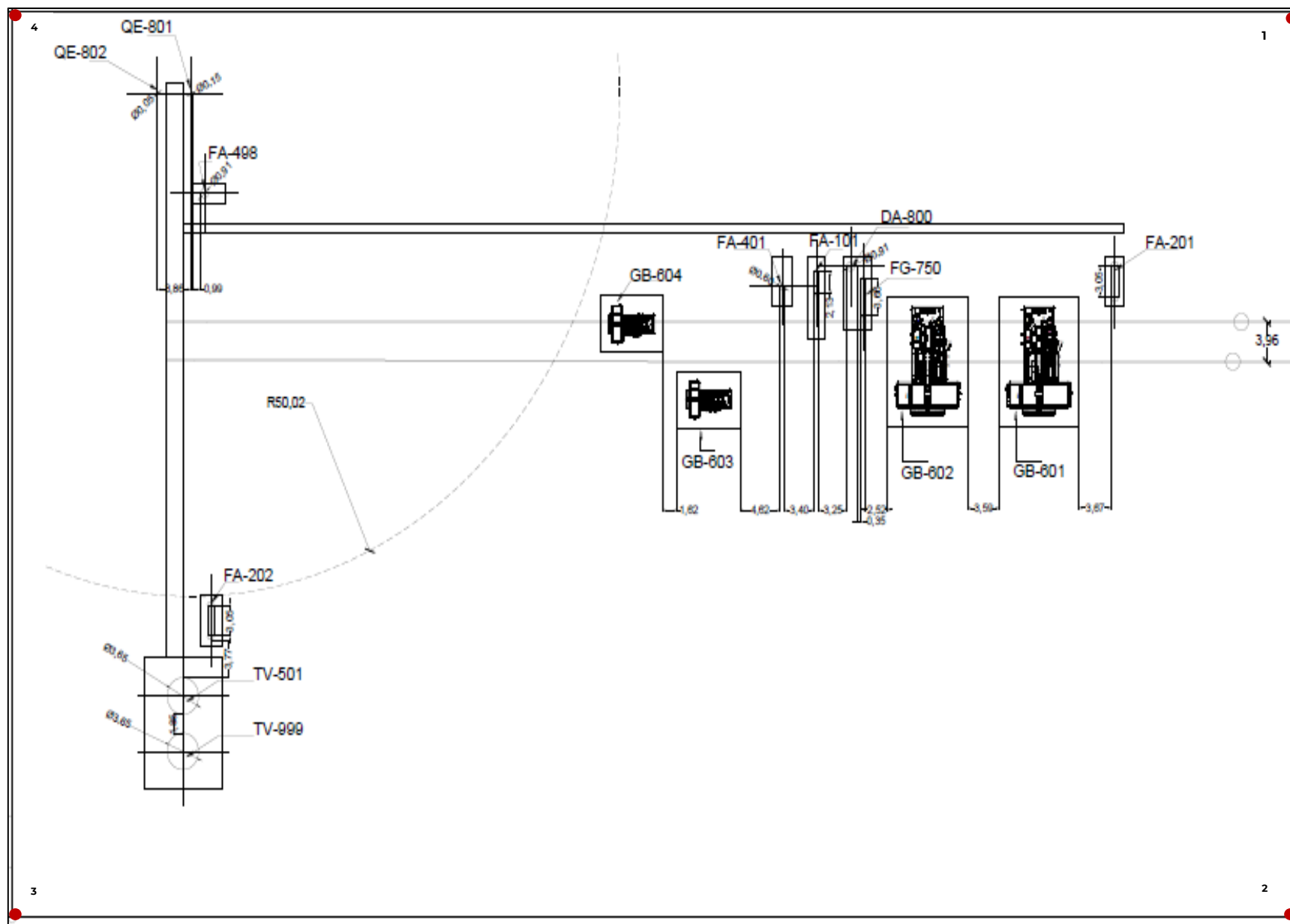
Figura 11 Lay-out del arreglo de equipos de la Planta de Acondicionamiento de Gas Natural.
