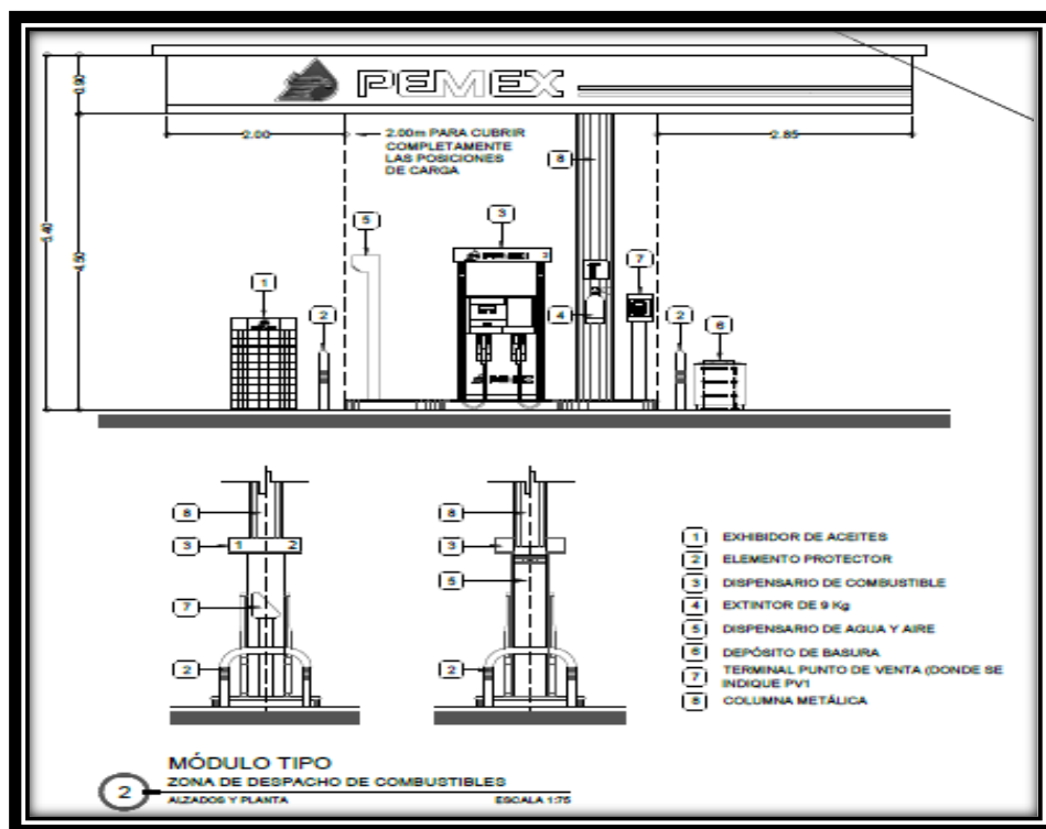
Imagen 10. Diagrama Tipo del Módulo de Abastecimiento
