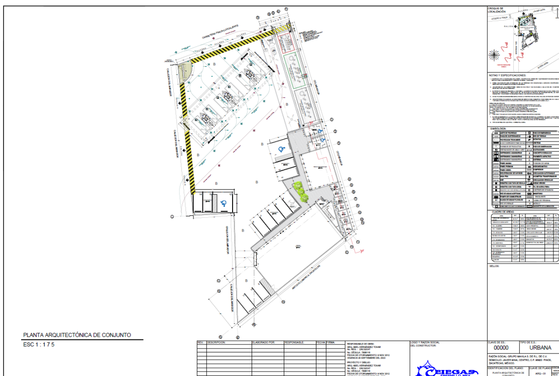
Imagen 35. Plano de Conjunto de la estacion de servicio.
