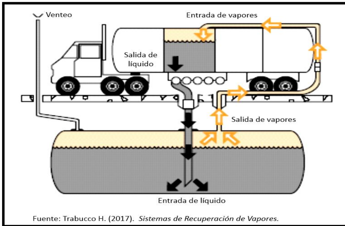
Ilustración 9. Sistema de recuperación de vapores Fase I.
