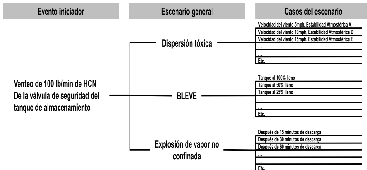
Figura IV.10.- Árbol de eventos para la fuga de ácido cianhídrico.
