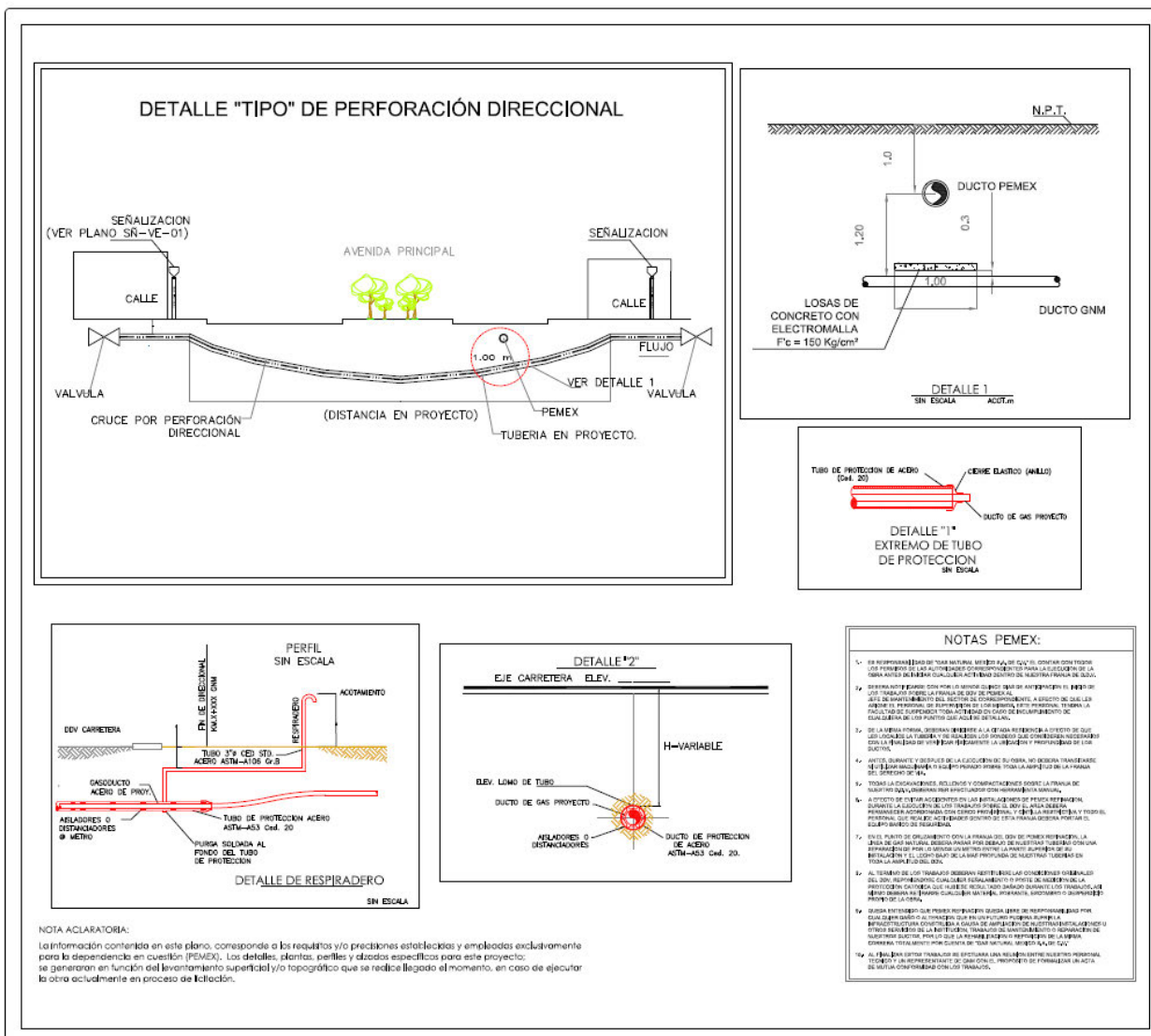
Figura II.4.- Cruce con ducto de PEMEX.
