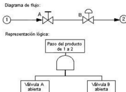
Figura IV.7.- Ejemplo de uso de la puerta lógica “Y” y su árbol de fallos.
