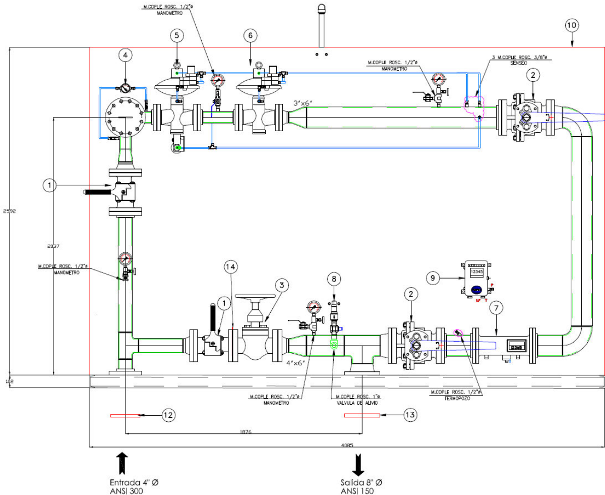
Figura II.5.- Componentes principales de una estación de regulación y medición.
