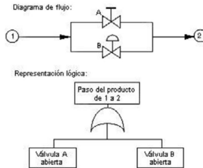
Figura IV.6.- Ejemplo de uso de la puerta lógica “O” y su árbol de fallos.
