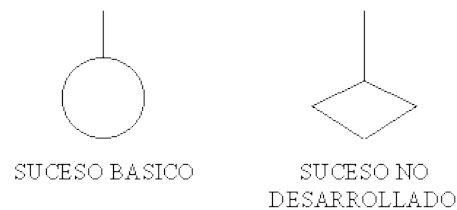
Figura IV.8.- Representación de los sucesos no desarrollados o básicos en el árbol de fallos.
