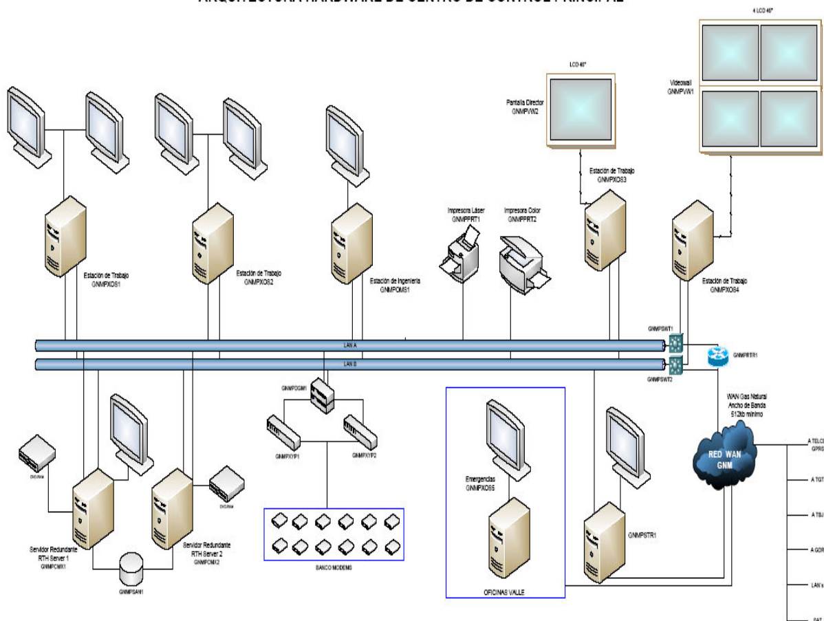
Figura II.6.- Diagrama del Cetro de Control de Distribución.
