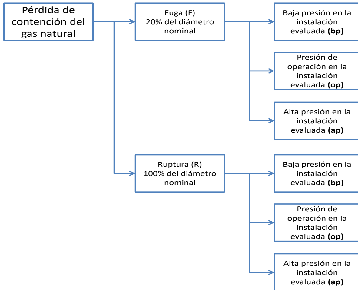
Figura IV.13.- Árbol de eventos para el escenario de pérdida de contención de gas natural en la red de distribución del PROYECTO que se presenta.
