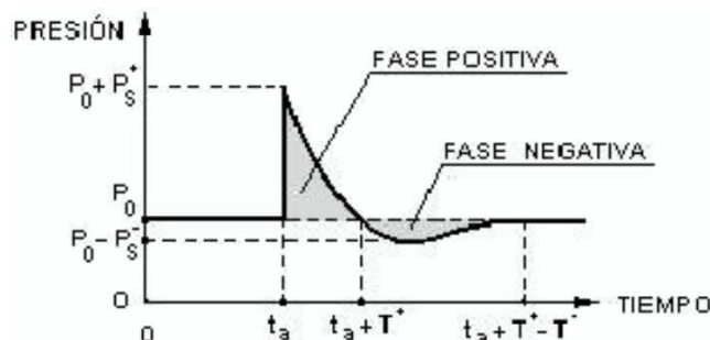
Figura IV.12.- Nivel de sobrepresión v.s. tiempo en una explosión.
