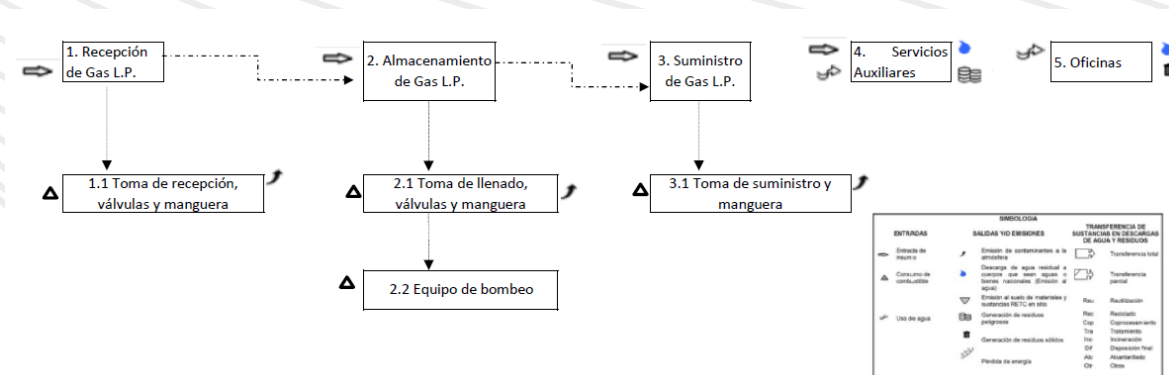
Ilustración 14. Diagrama de gas LP
