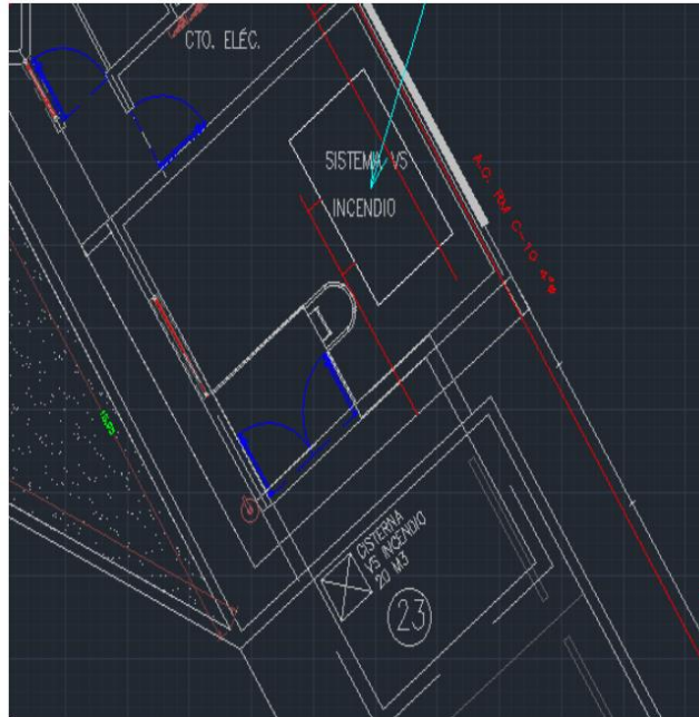
Ilustración 8. Ubicación de Cisterna y Cuarto de maquinas
