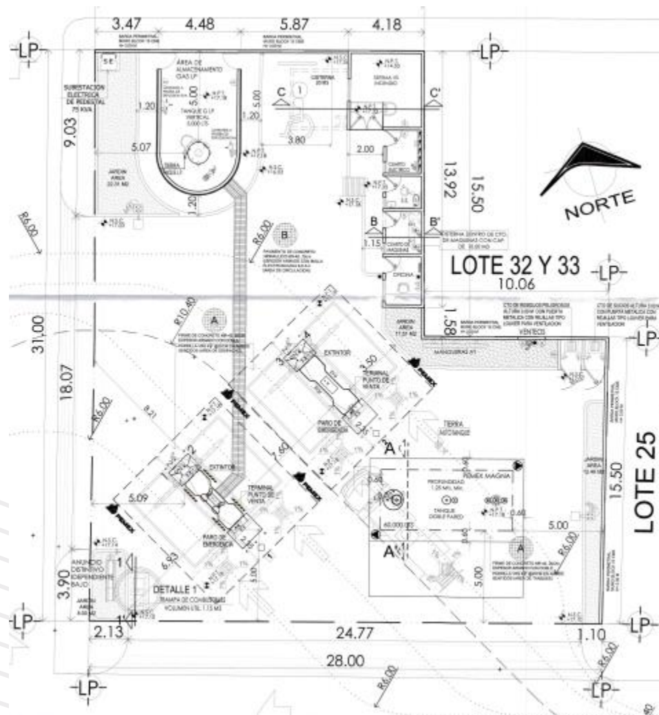
Ilustración 13. Plano del proyecto
