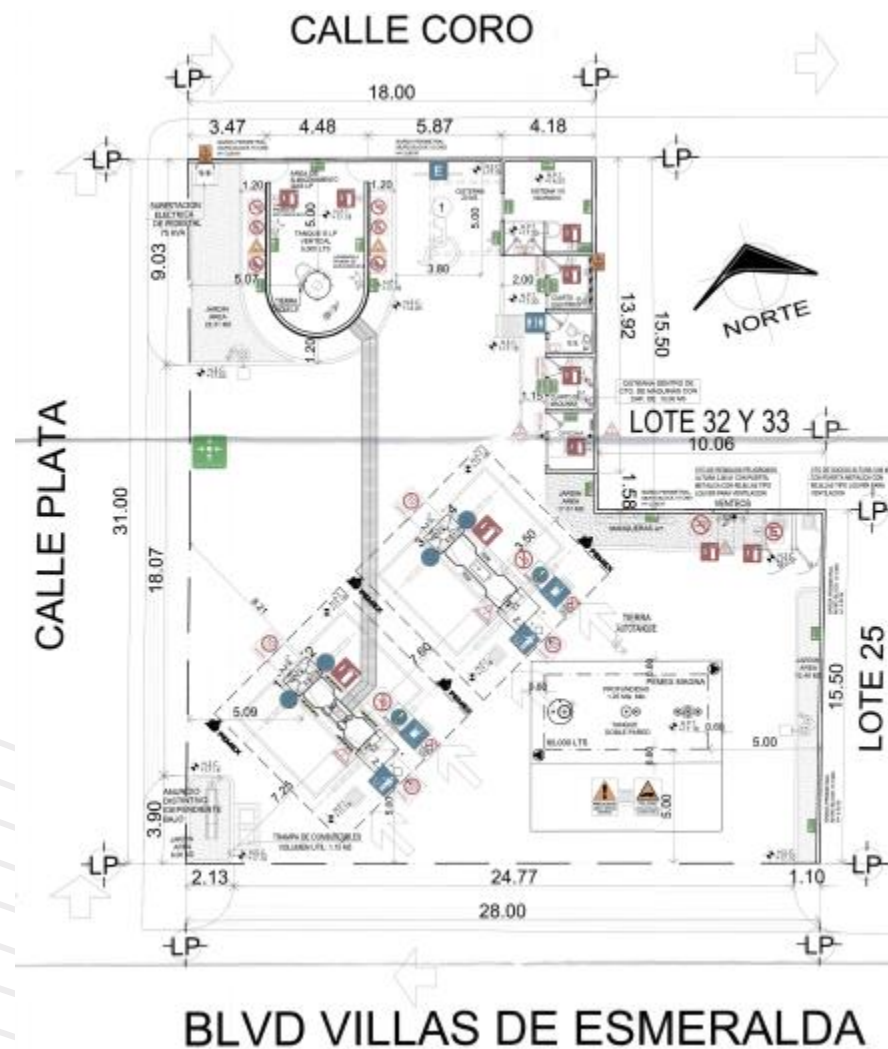
Ilustración 10. Trayectoria de hidrantes
