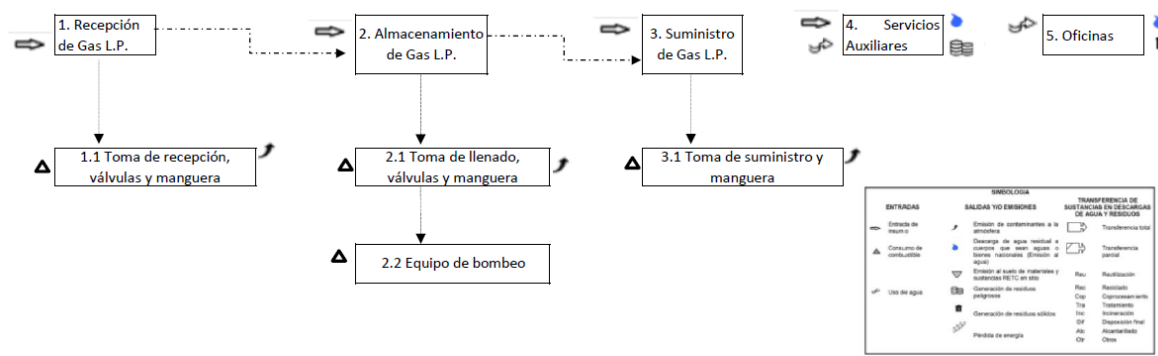
Ilustración 17. Diagrama de gas LP
