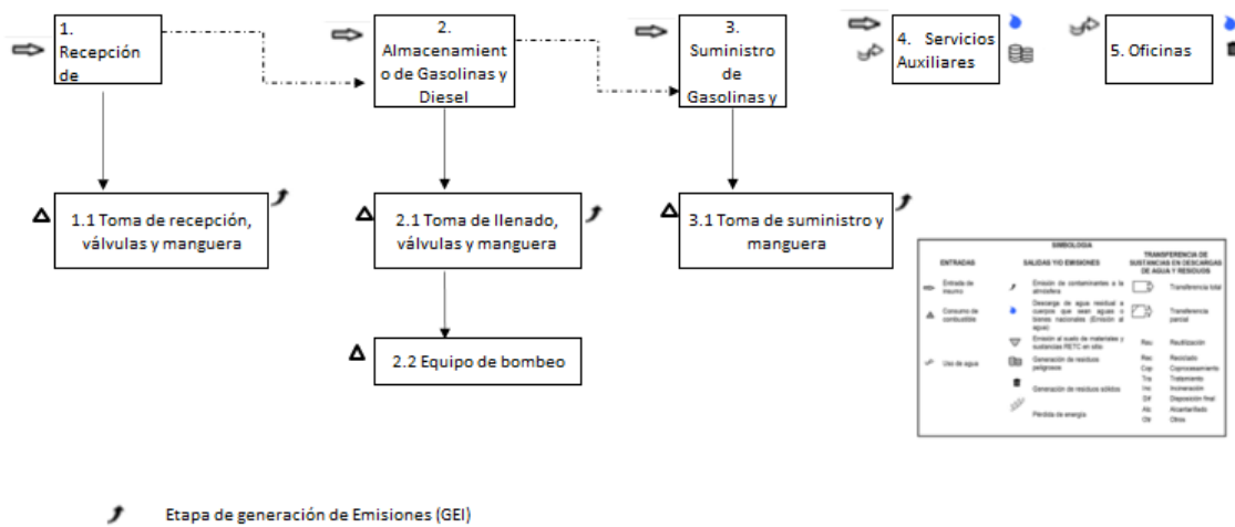
Ilustración 18. Diagrama gasolinas
