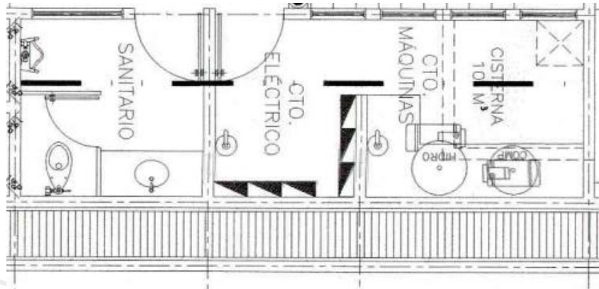
Ilustración 9. Ubicación de Cisterna y Cuarto de maquinas
