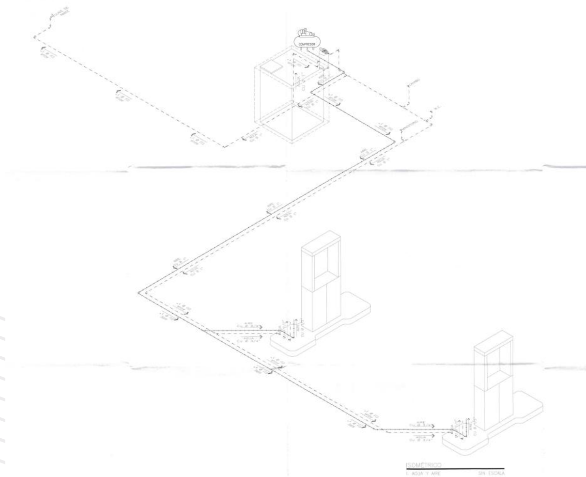
Ilustración 10. Trayectoria de hidrantes
