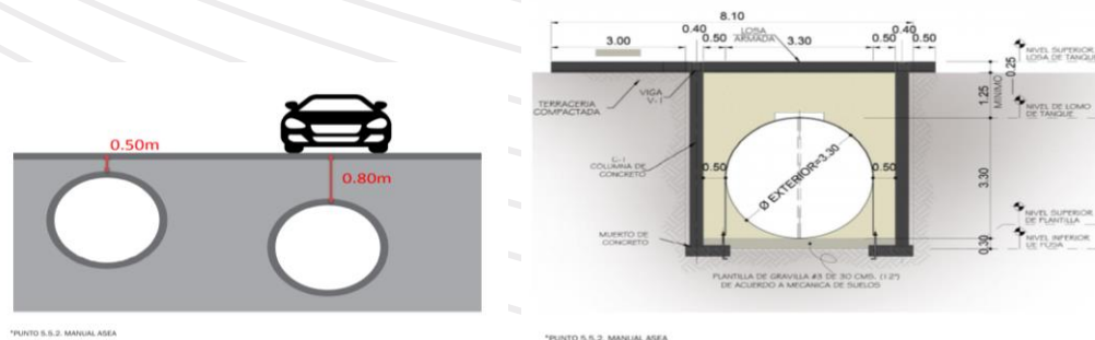
Ilustración 14 Fosa de recipientes de almacenamiento de Gasolinas
