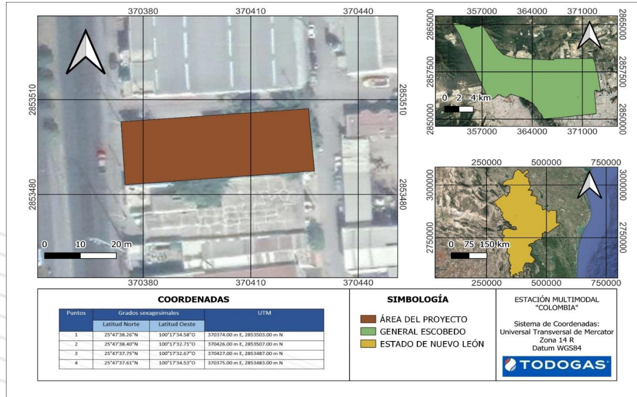
Ilustración 11. Representación Regional del proyecto
