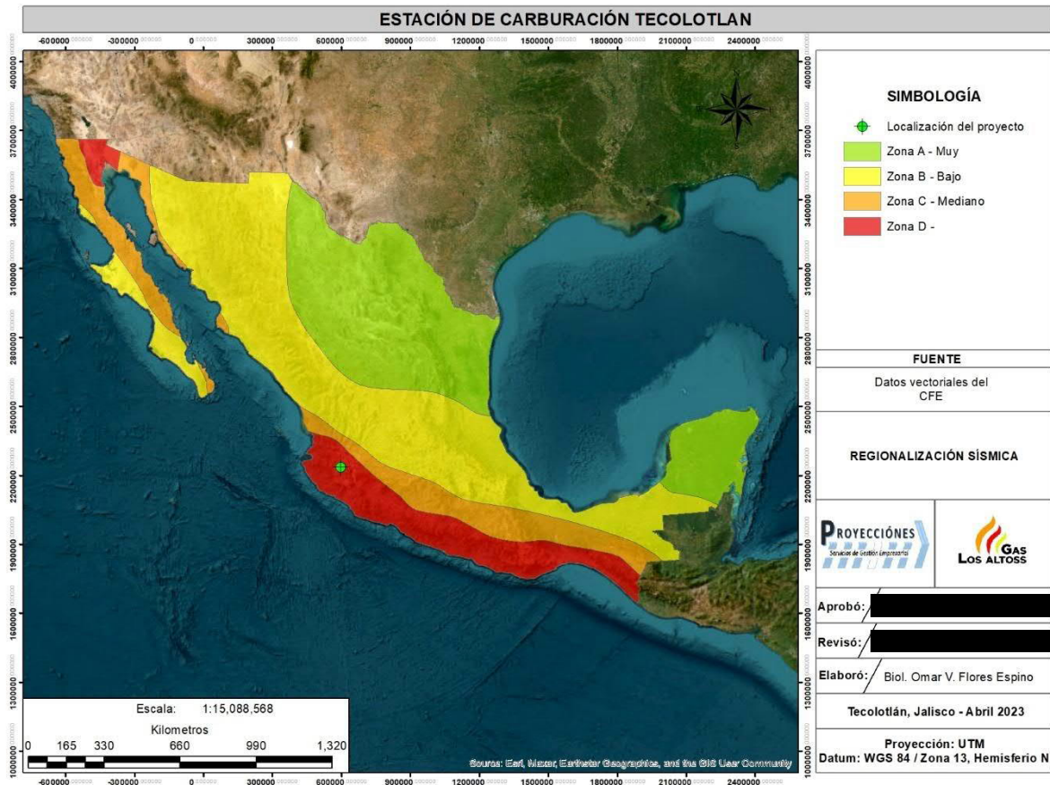
Figura 6. Regionalización sísmica.
