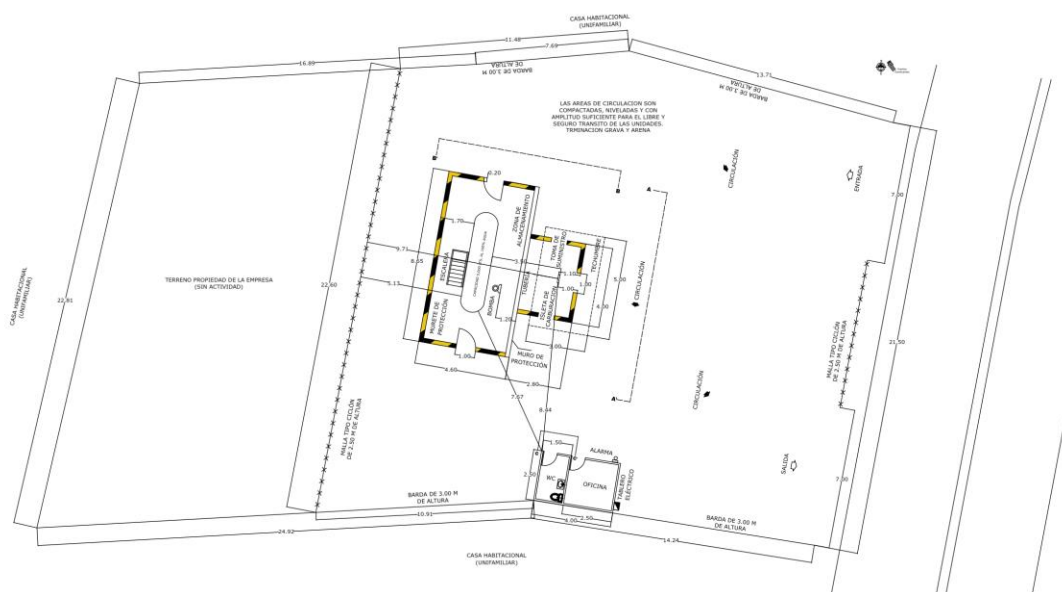
Figura III.1.b)-2. Plano Proyecto Civil
