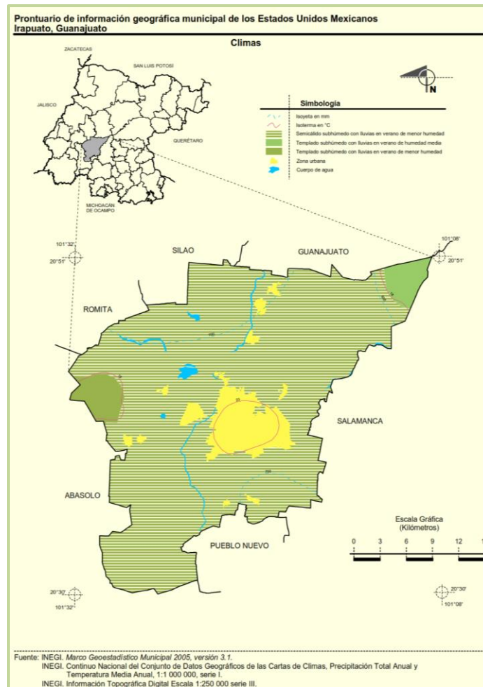
Figura III.4.d)-A1. Clima
