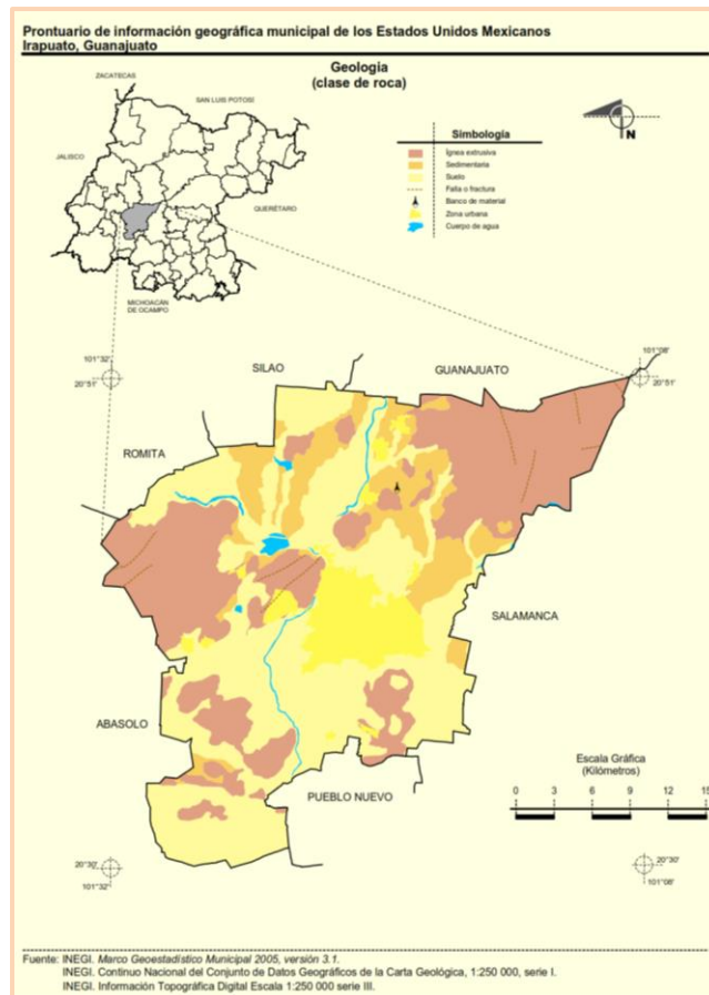
Figura III.4.d)-B1. Geología
