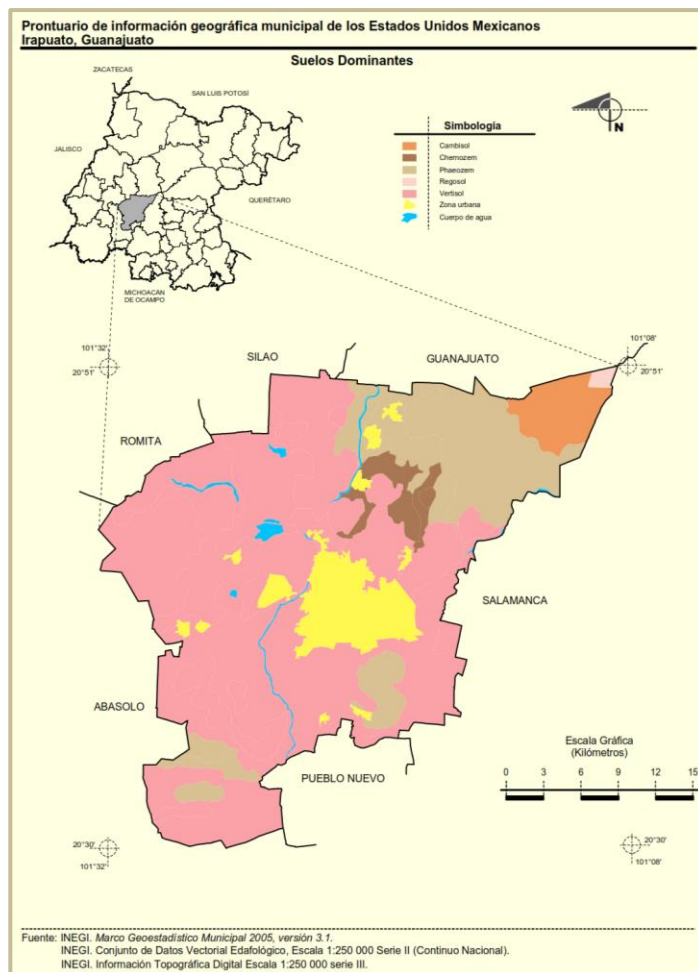
Figura III.4.d)-C1. Suelos
