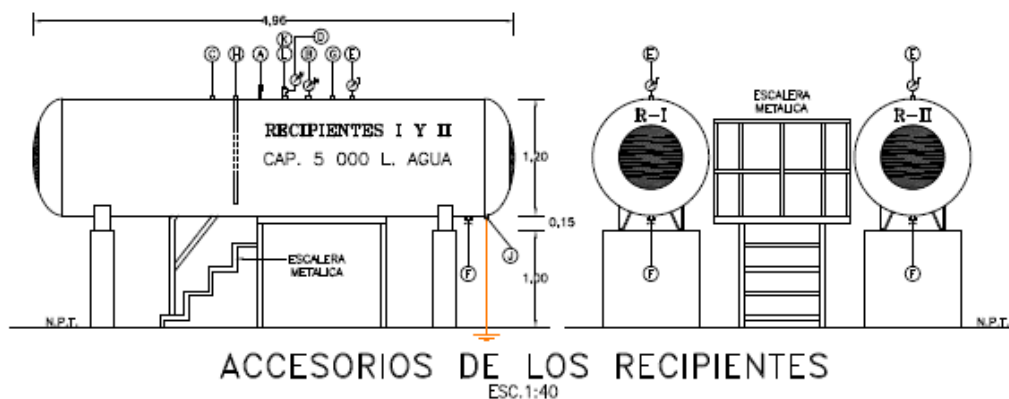
Figura 9. Instrumental de seguridad de los tanques de almacenamiento.
