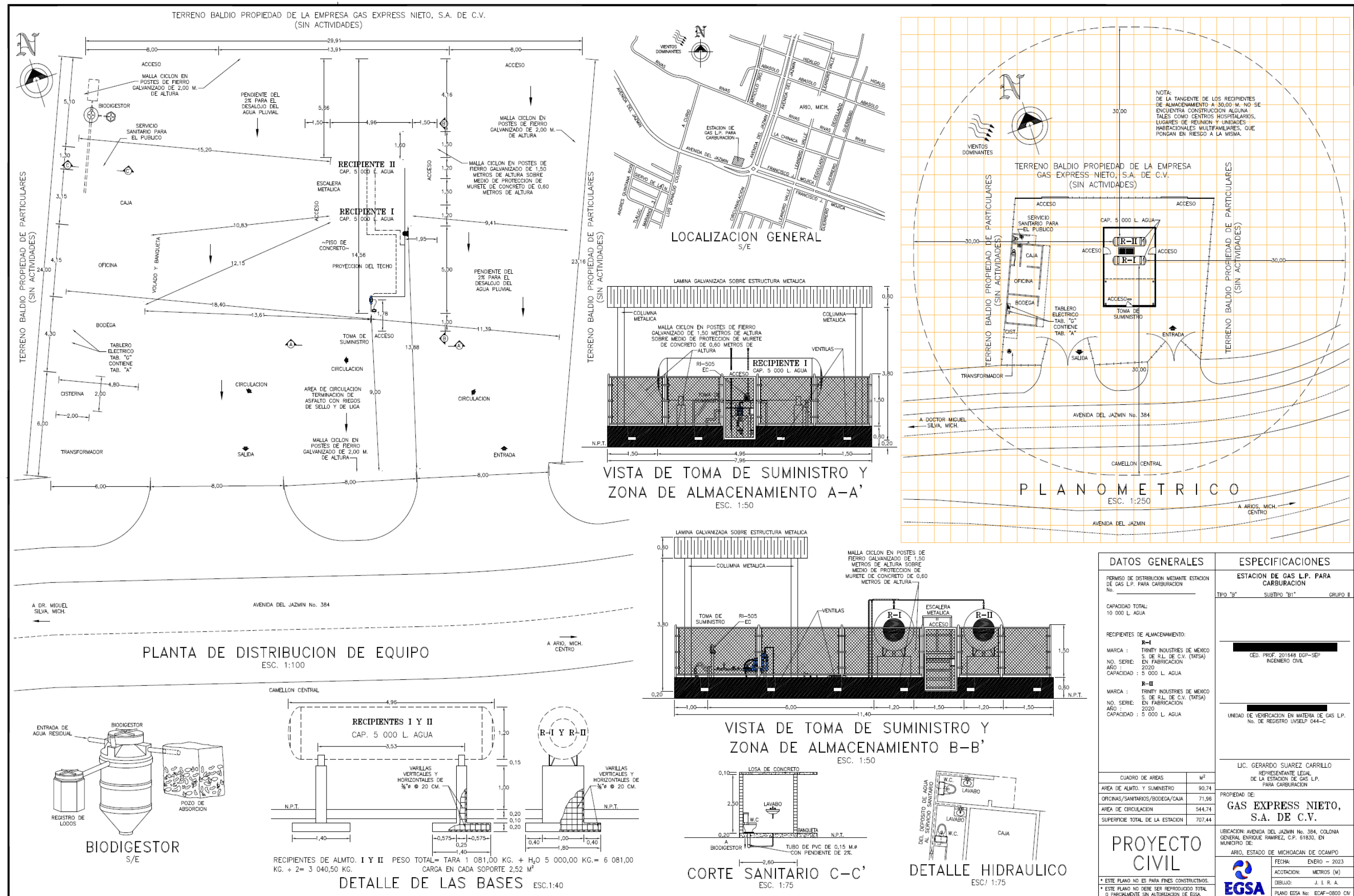
Figura 4. Plano de arreglo general de áreas en la sección de terreno seleccionado para el proyecto.
