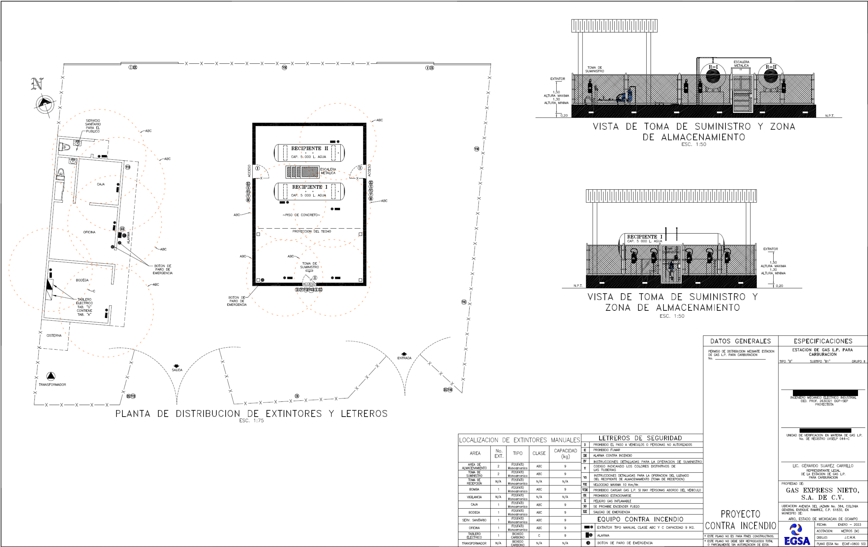
Figura 17. Se observa el plano de instalaciones de seguridad proyectadas para las instalaciones de la estación.
