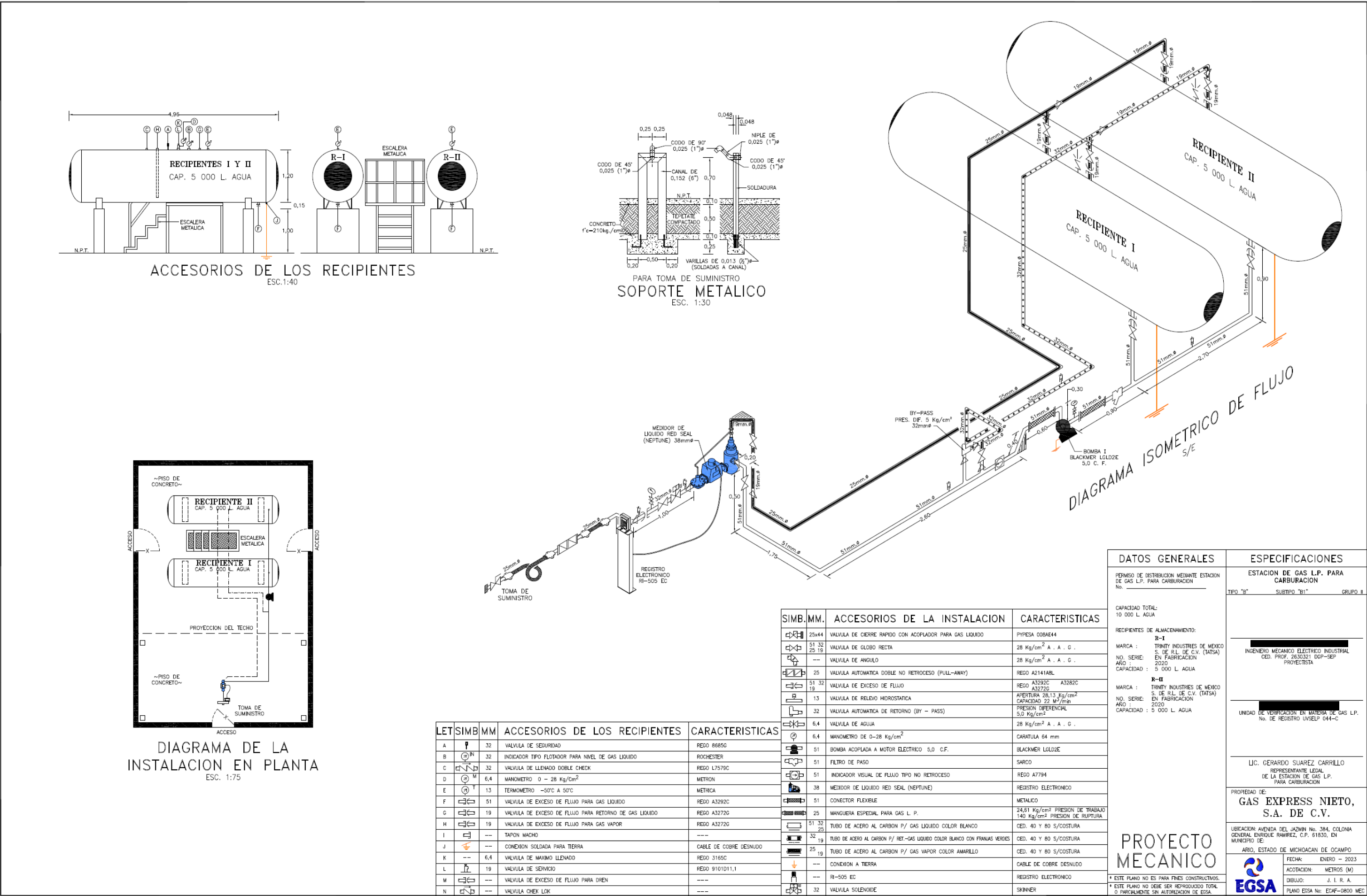
Figura 5. Plano de arreglo mecánico con detalles de equipamiento dentro de la estación proyectada.
