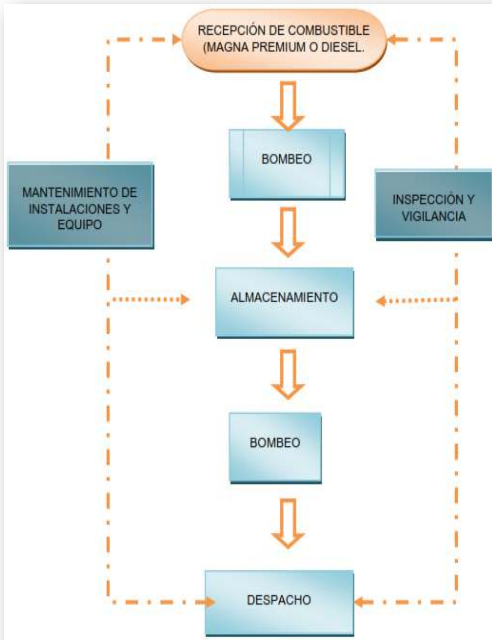
Figura 4. Diagrama de bloques de la operación de la estación de servicio
