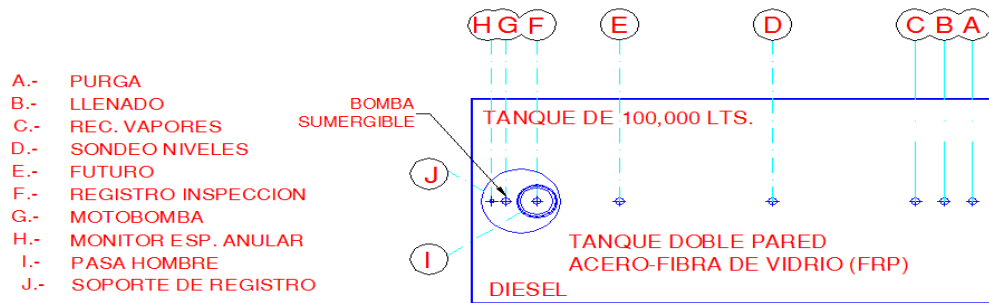
Figura 10: Dispositivos de seguridad con los que contarán los tanques de almacenamiento.
