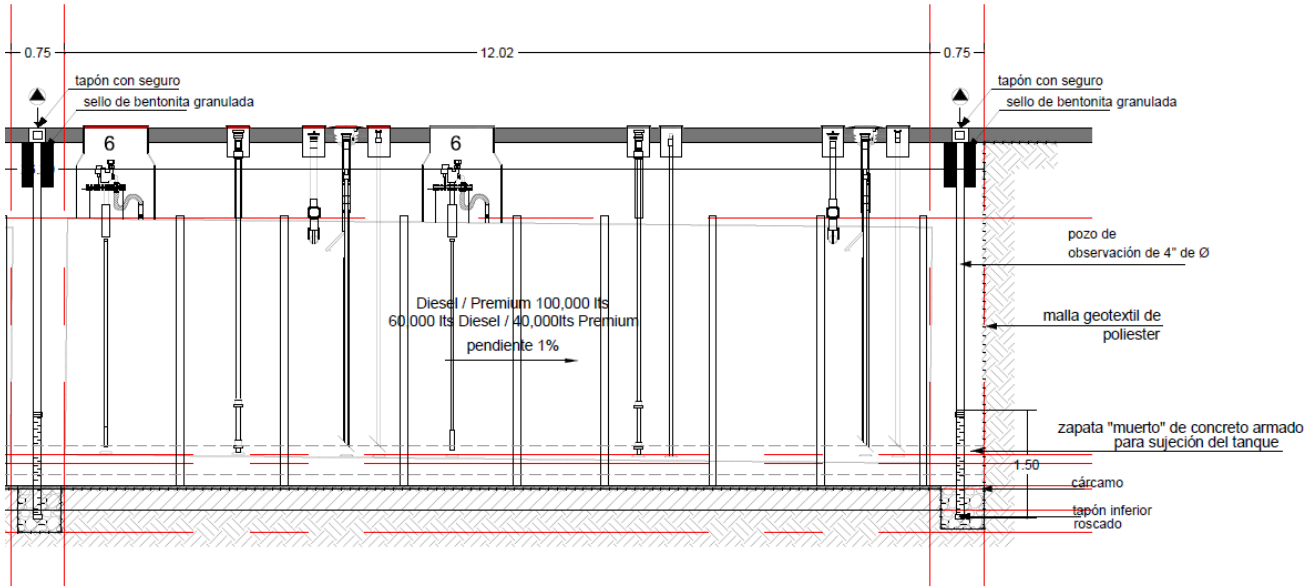
Figura 9: Accesorios con los que contarán los tanques de Almacenamiento.
