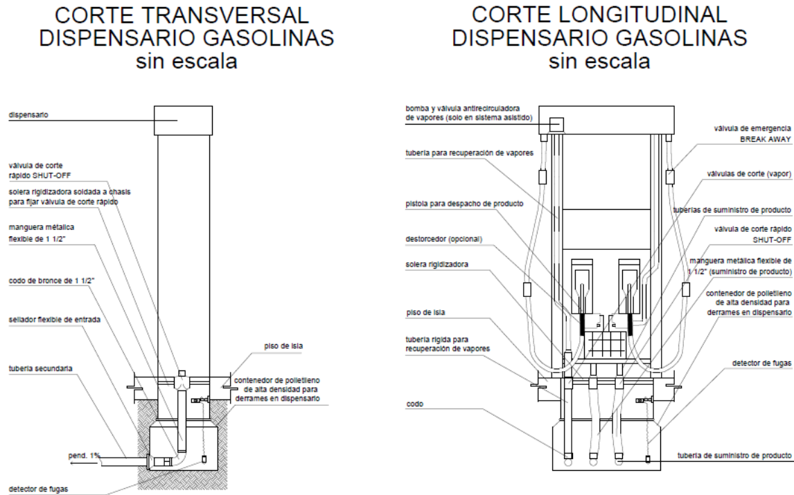
Figura 11: Componentes de los dispensarios de la Estación.
