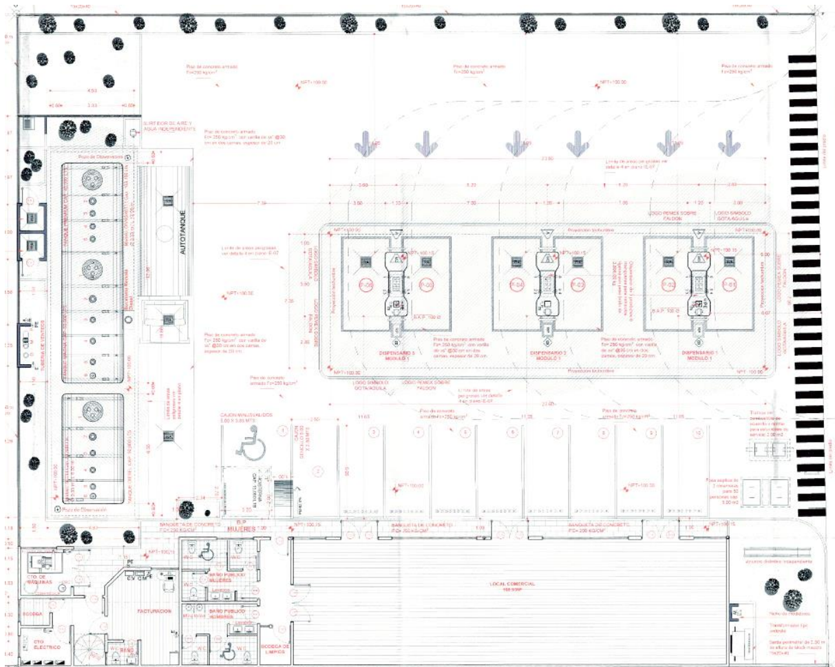
Imagen 12. Plano de Conjunto de ESTACION DE SERVICIO, "SALPAT COMBUSTIBLES S.A. DE C.V."
