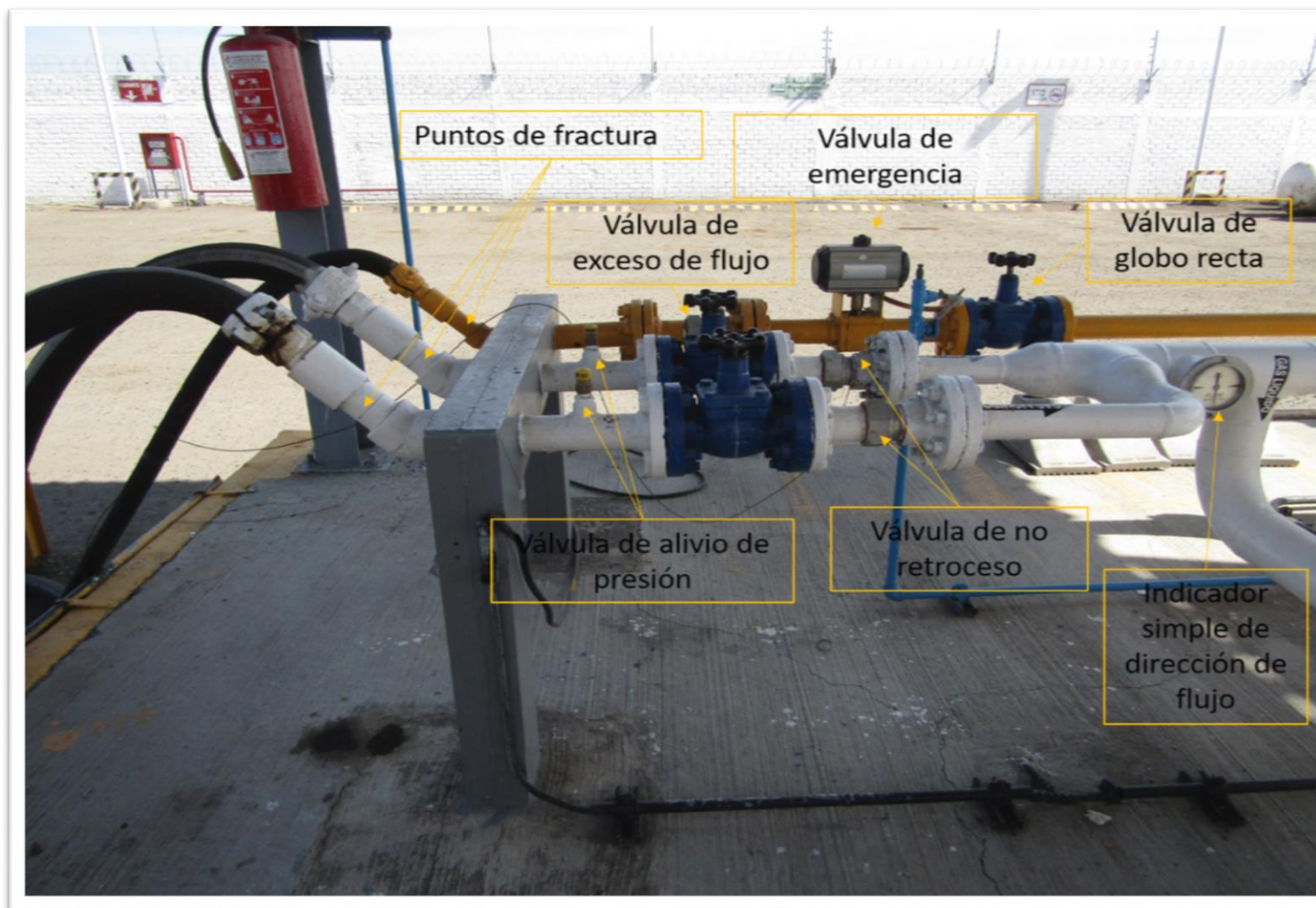
Figura IV.3: Equipos de seguridad en las tomas de recepción.
