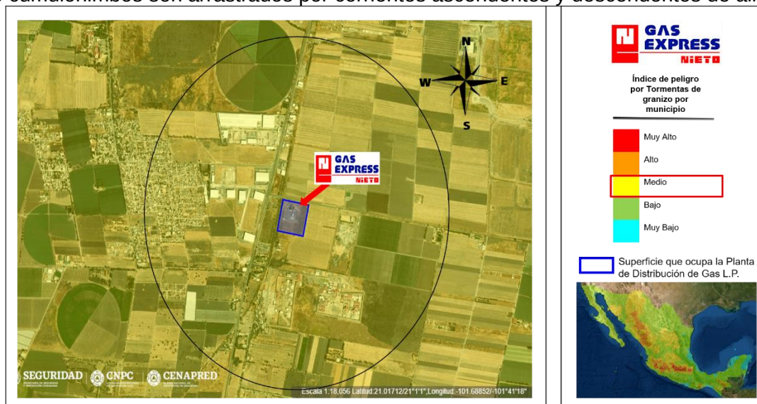
Figura II. 13: Peligro por tormentas por granizo.
