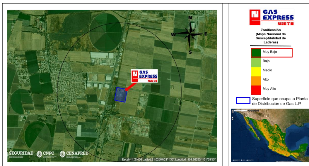
Figura II. 7: Peligro por susceptibilidad por laderas. Fuente: Atlas Nacional de Riesgos.
