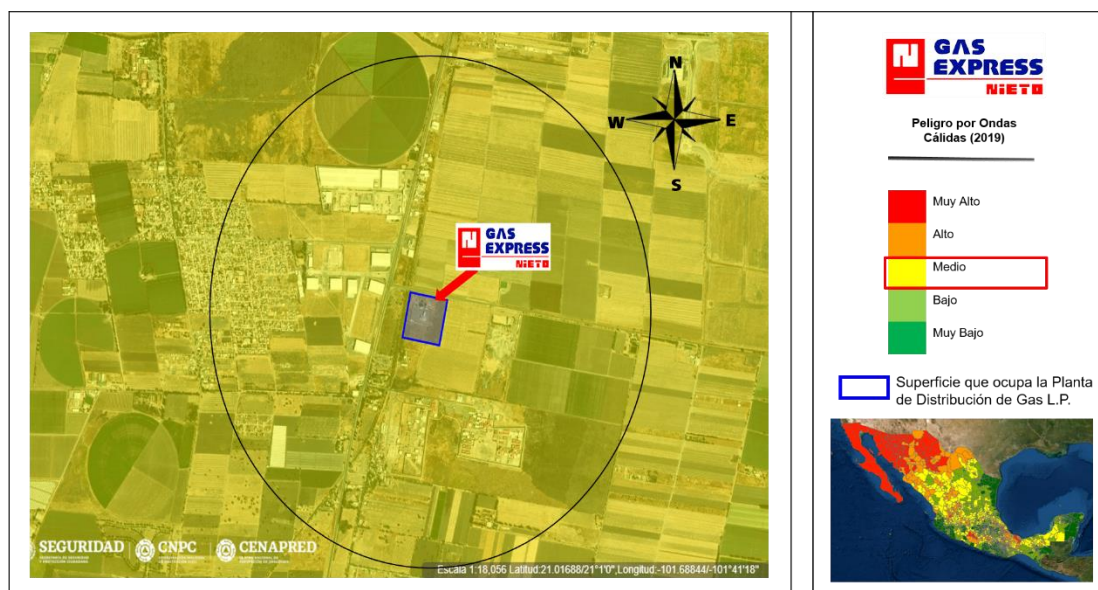
Figura II. 15: Peligro por ondas cálidas. Fuente: Ondas cálidas, Atlas Nacional de Riesgos.
