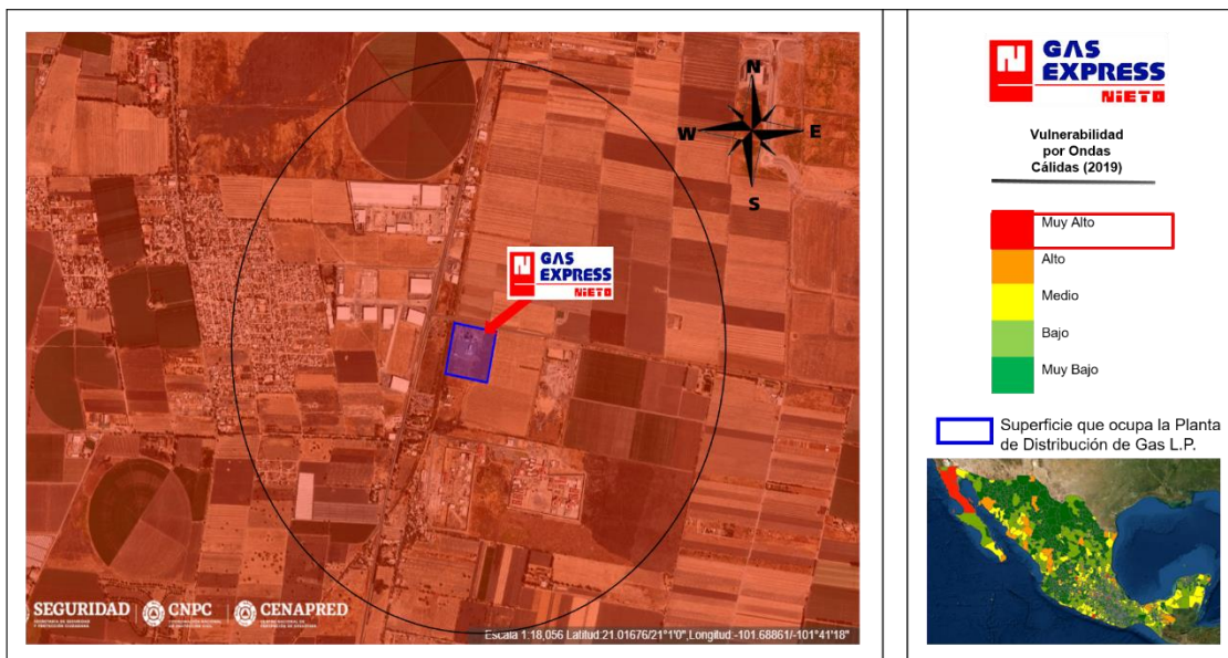
Figura II. 14: Vulnerabilidad por ondas cálidas. Fuente: Ondas cálidas, Atlas Nacional de Riesgos.
