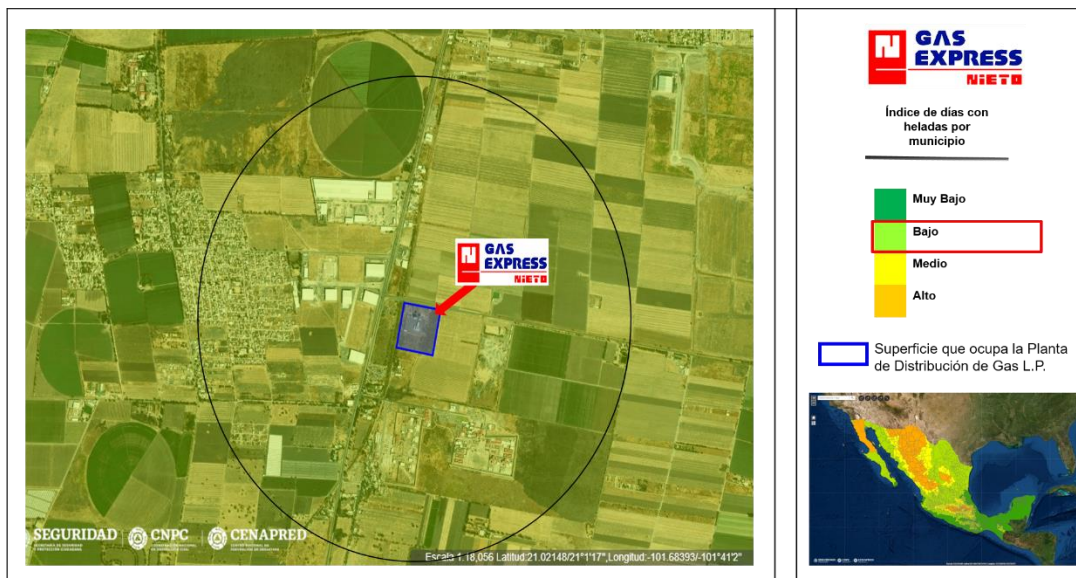
Figura II. 16: Índice de días con heladas. Fuente: Atlas Nacional de Riesgos.
