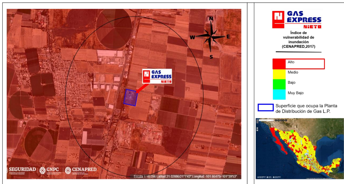
Figura II. 8: Índice de vulnerabilidad por inundación. Fuente: Inundación, CENAPRED, 2017
