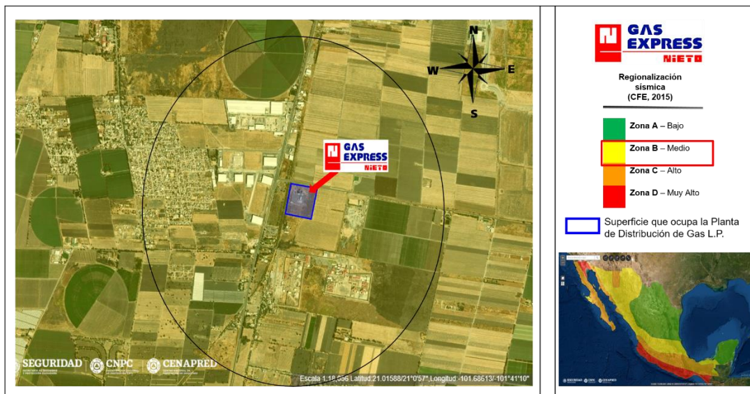
Figura II. 6: Regionalización sísmica. Fuente: Regionalización sísmica, CFE 2015, CENAPRED.
