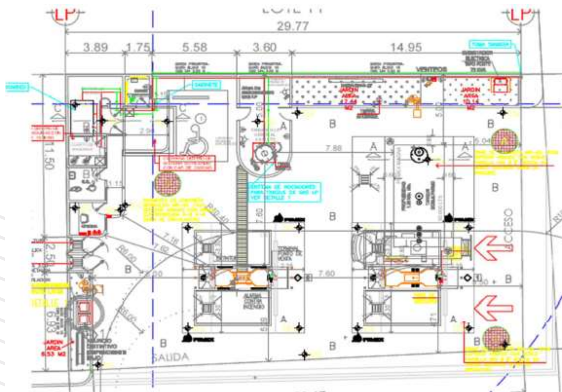
Ilustración 13. Plano de Trayectorias Proyecto Contra Incendio
