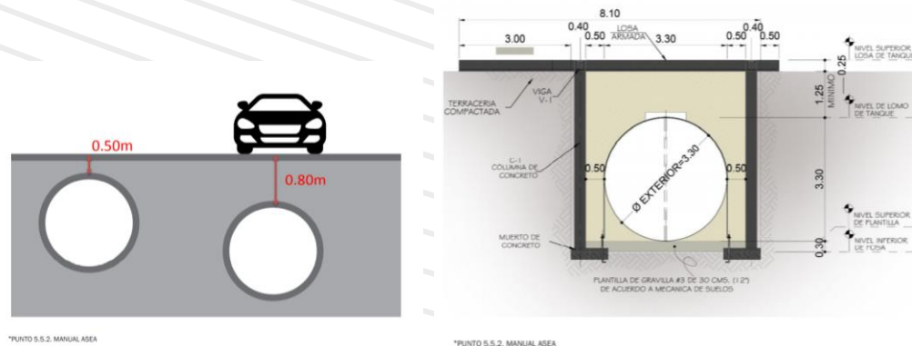
Ilustración 15 Fosa de recipientes de almacenamiento de gasolinas y diésel
