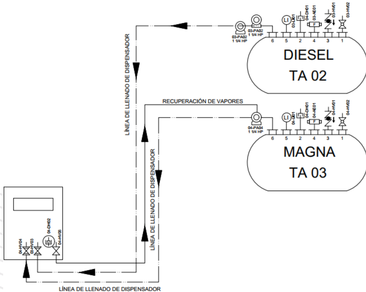
Ilustración 10. El sistema de tuberías para la conducción de combustibles líquidos
