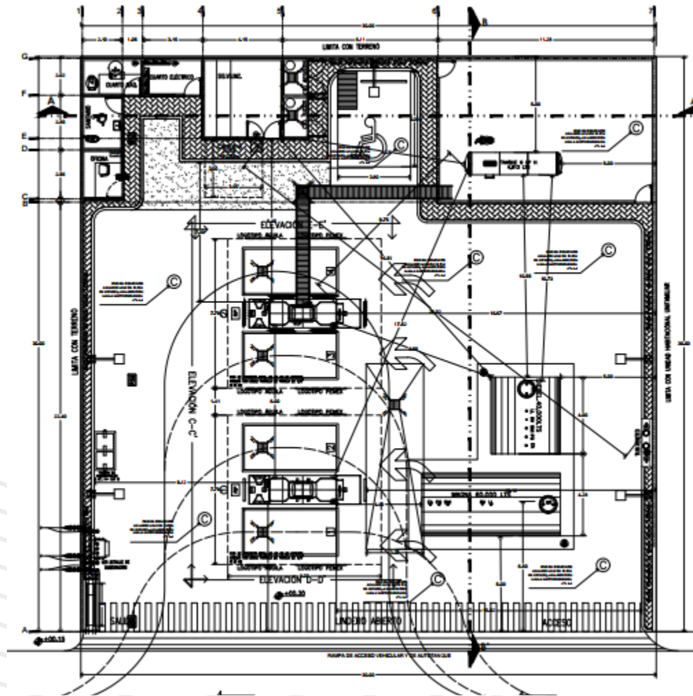
Ilustración 14. Plano del proyecto
