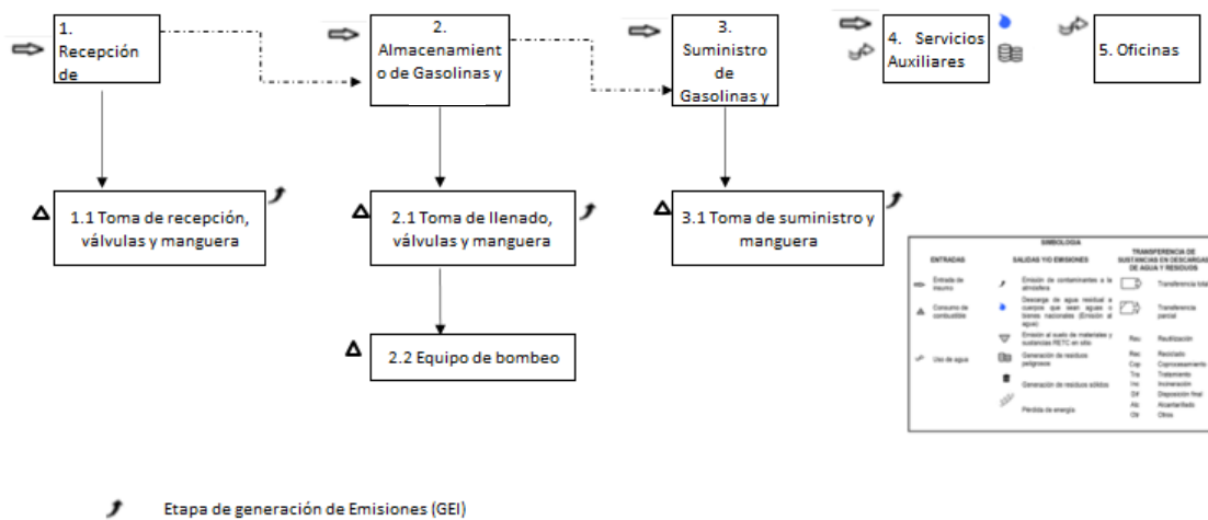
Ilustración 18. Diagrama gasolina / Diésel
