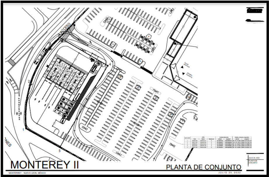
Figura 9. Sembrado de la Estación de Servicio dentro del predio de la Tienda COSTCO MONTERREY.
