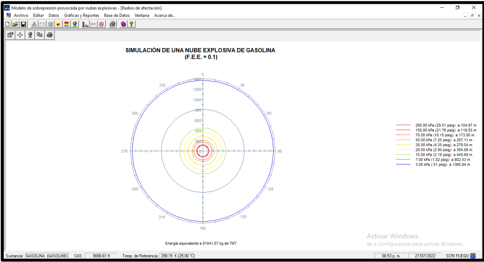
Figura 13. Simulación de máximo catastrófico.
