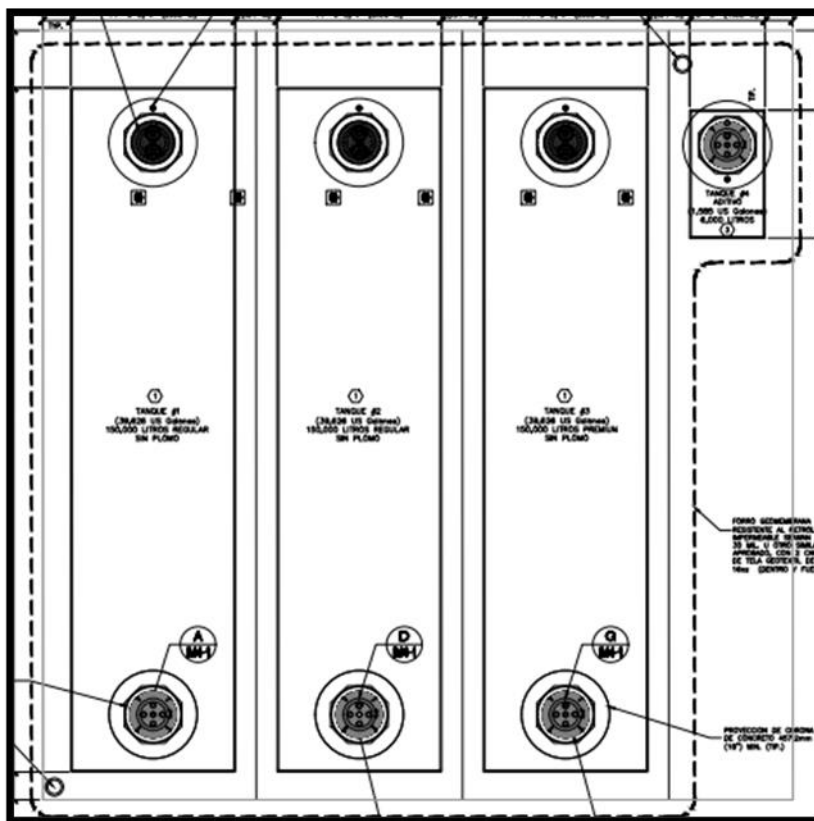
Figura 16. Tanques subterráneos doble pared de acero / polietileno.
