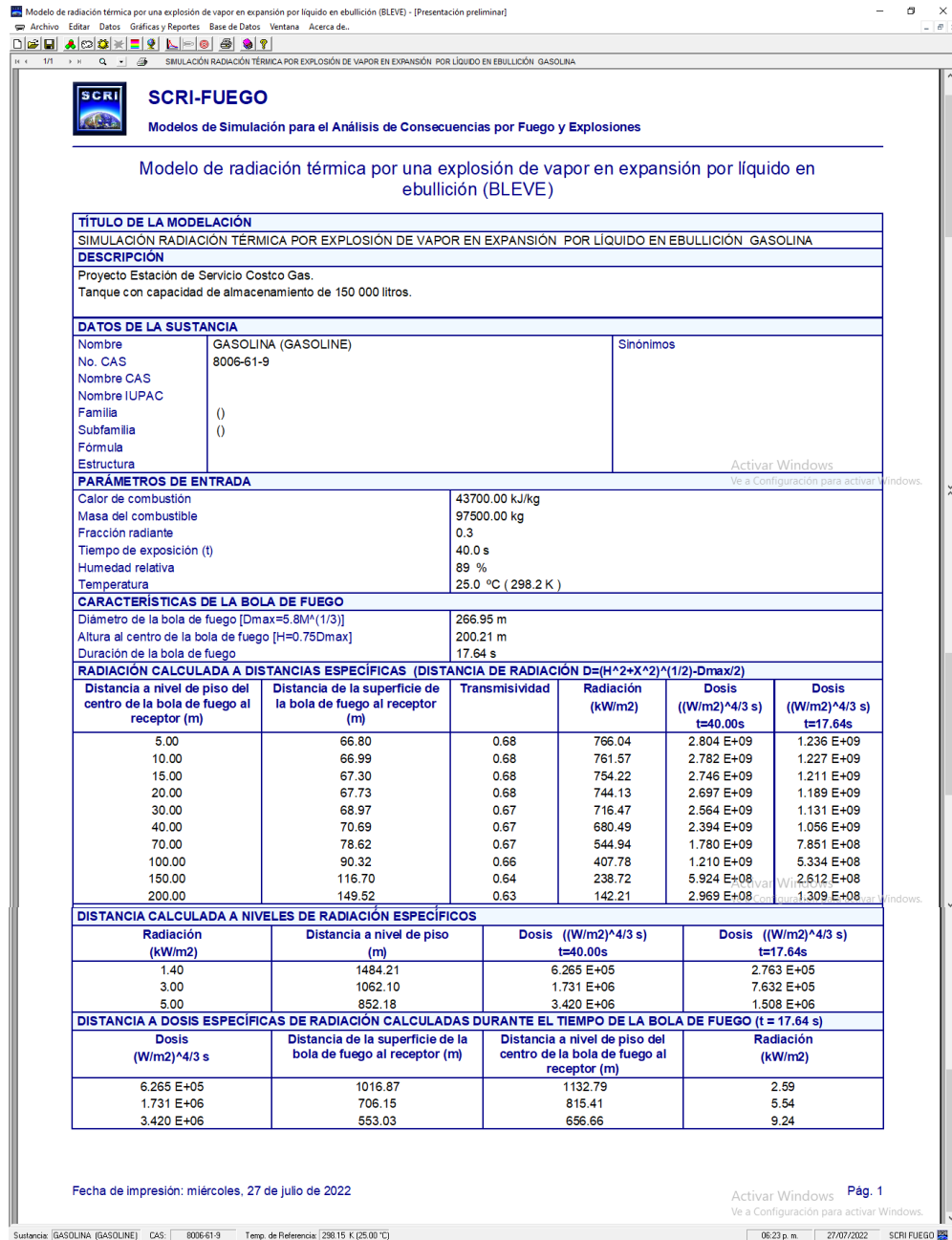
Figura 14. Simulación de máximo catastrófico.
