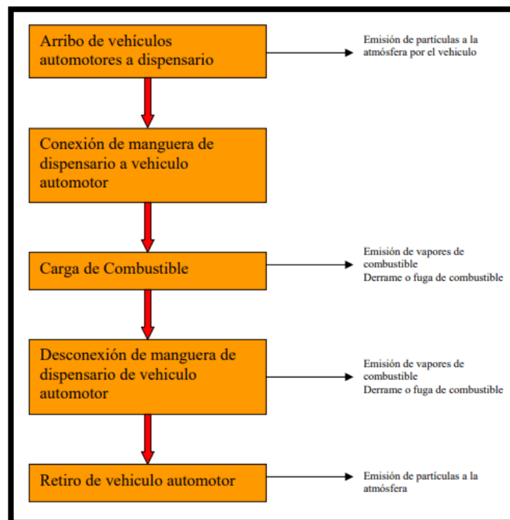
Figura 19. Flujograma de proceso de carga de combustible a usuarios y emisión de contaminantes.
