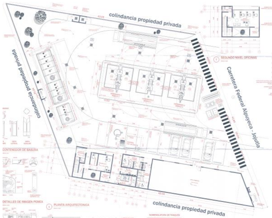
Imagen 37. Plano de Conjunto de la estacion de servicio.
