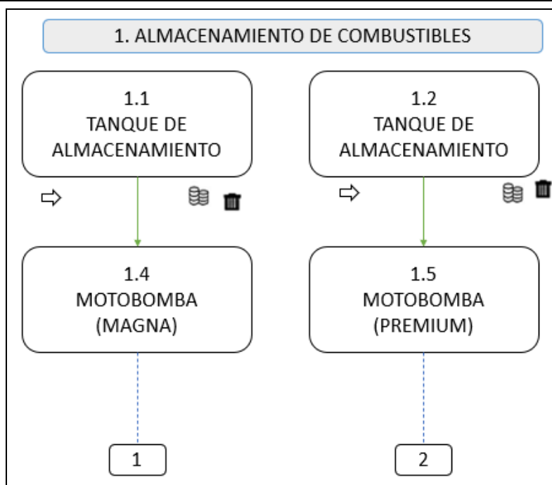
Figura 10. Almacenamiento de combustibles.
