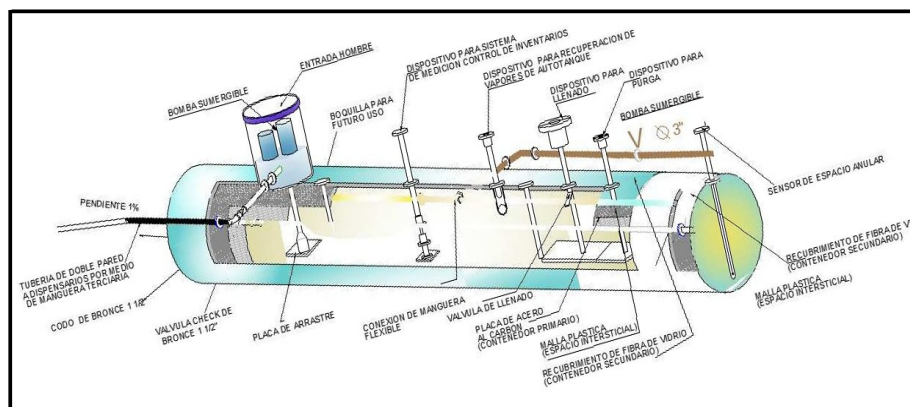
Corte esquemático de tanque de doble pared ecológico.
