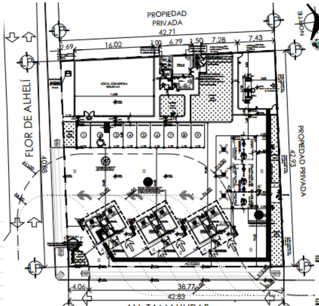
Ilustración 15. Plano del proyecto
