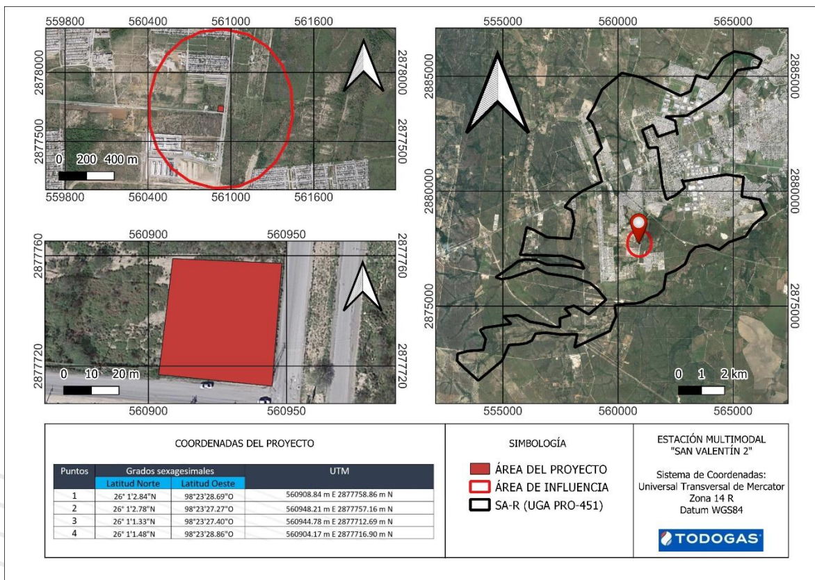
Ilustración 24. Sistema Ambiental Regional, Área de Influencia y Área del Proyecto
