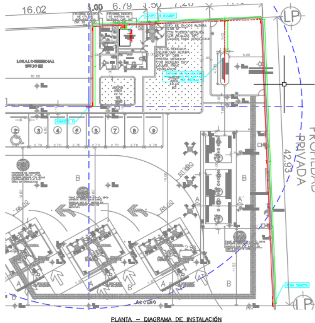
Ilustración 12. Trayectoria de hidrantes
