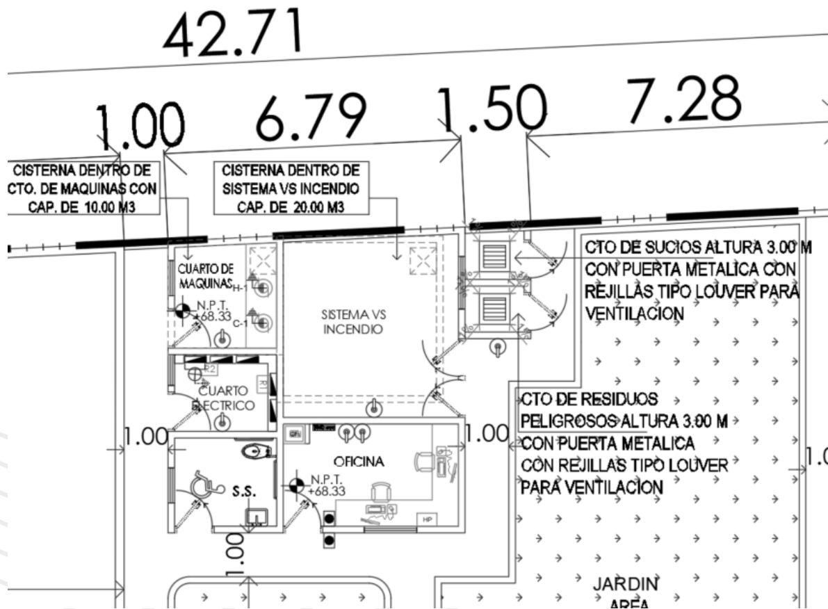
Ilustración 11. Ubicación de Cisterna y Cuarto de máquinas
