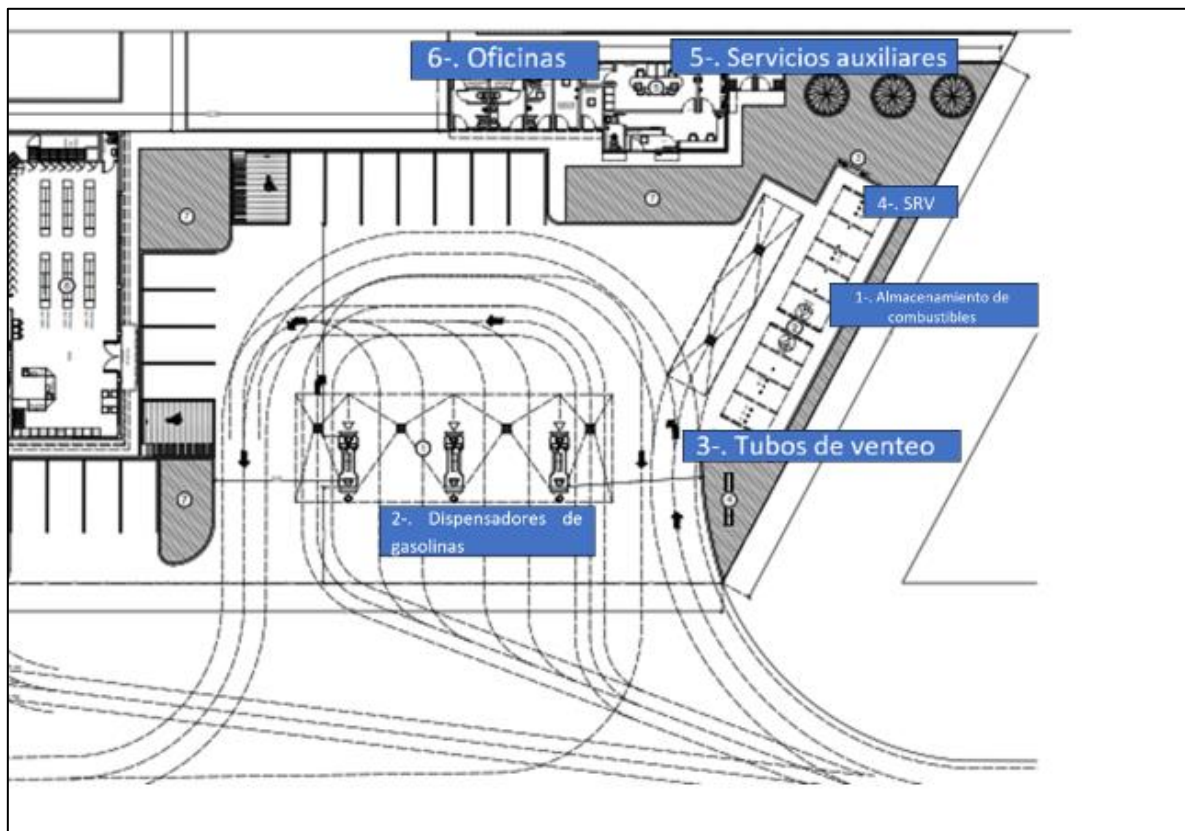
Figura 11. Diagrama de plano de la Estación de servicio que pretende establecerse.
