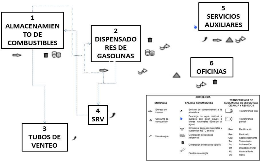
Figura 12. Diagrama de funcionamiento general para la Estación de Servicio.
