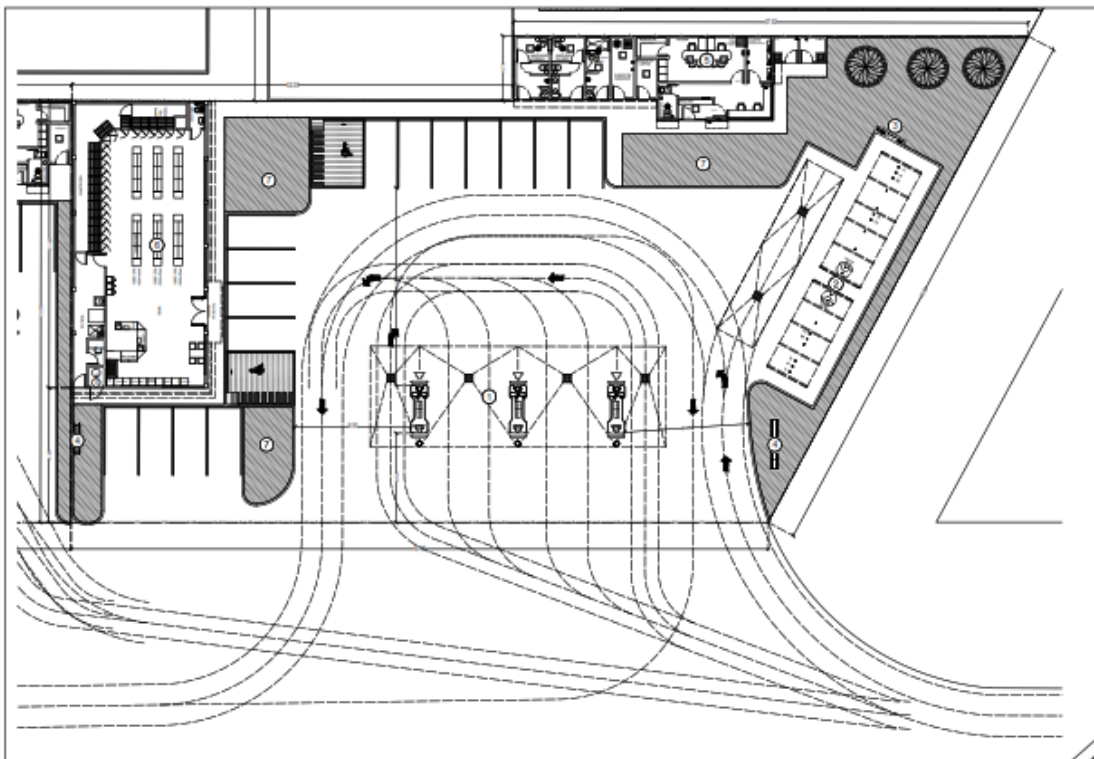
Figura 3. Plano de la estación de servicio.
