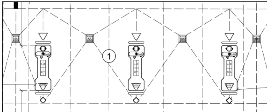
Figura 8. Área de dispensarios en la estación de servicio.
