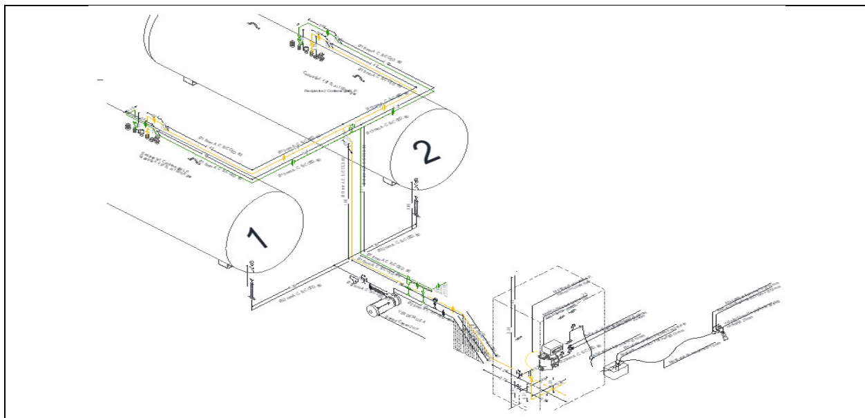
FIGURA III.1.3.6. DIAGRAMA ISOMÉTRICO DE LA INSTALACIÓN DE ALMACENAMIENTO-IMPULSIÓN Y TRANSPORTE DE GAS LP EN LA ESTACIÓN | FUENTE: PLANO DEL PROYECTO MECÁNICO | ANEXO 3 EXPEDIENTE TÉCNICO DEL PROYECTO
