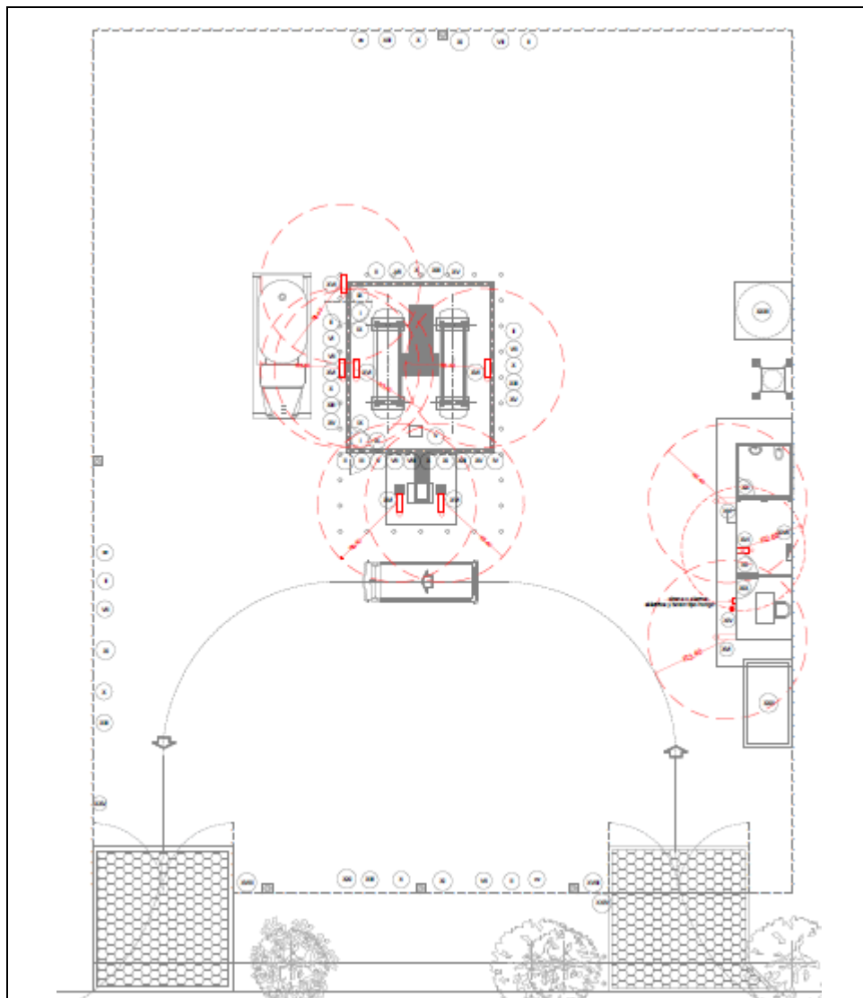
FIGURA III.1.3.8. DISTRIBUCIÓN DE EXTINTORES EN LA ESTACIÓN | FUENTE: PLANO DEL PROYECTO CONTRA INCENDIO ANEXO 3 EXPEDIENTE TÉCNICO DEL PROYECTO
