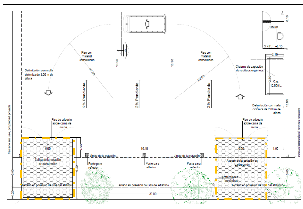
FIGURA III.1.3.1. ACCESO Y SALIDA A LA ESTACIÓN | FUENTE: PLANO DEL PROYECTO PLANOMÉTRICO | ANEXO 3 EXPEDIENTE TÉCNICO DEL PROYECTO
