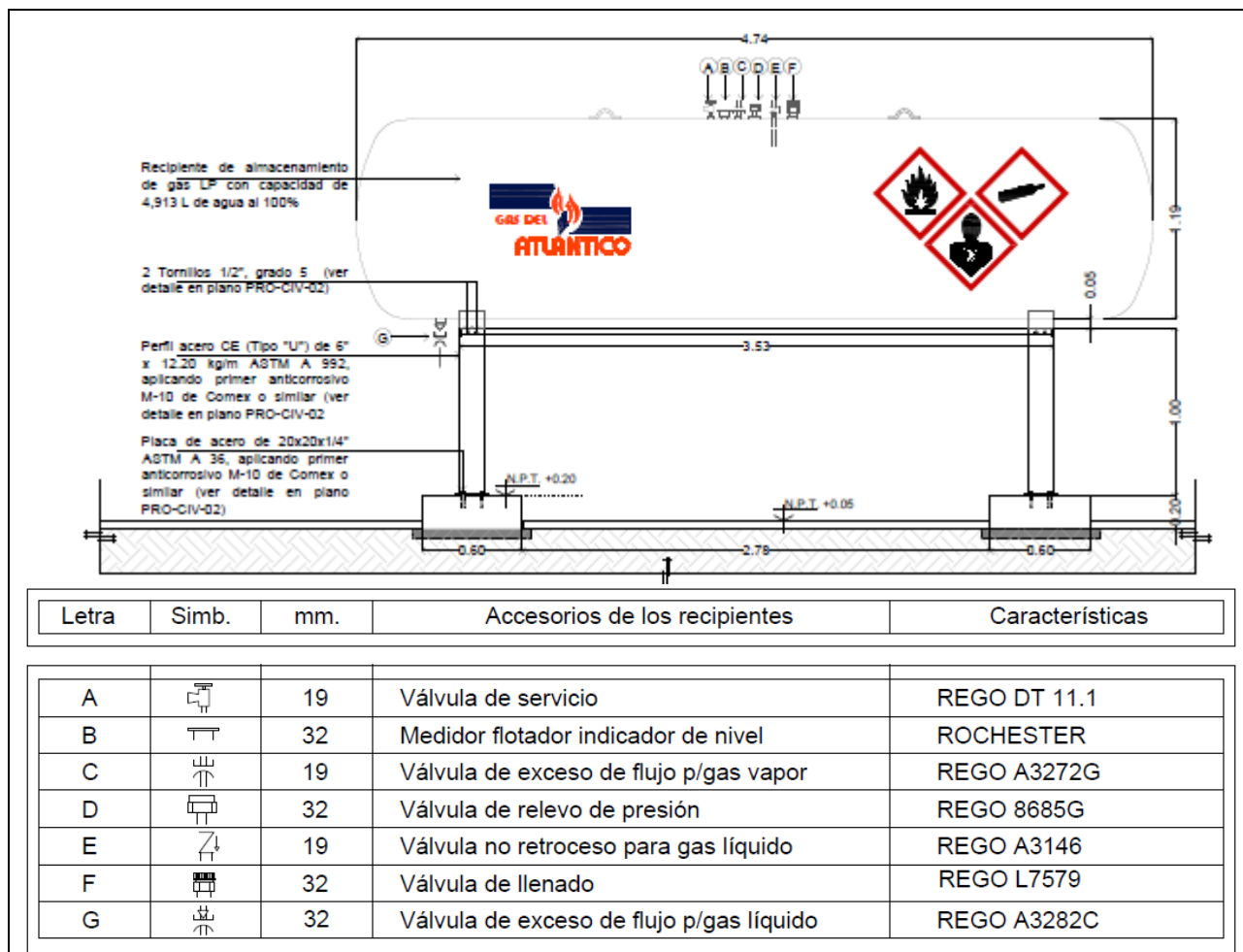
FIGURA III.1.3.4. LISTADO Y DISTRIBUCIÓN DE ACCESORIOS DEL TANQUE DE ALMACENAMIENTO FUENTE: PLANO DEL PROYECTO MECÁNICO | ANEXO 3 EXPEDIENTE TÉCNICO DEL PROYECTO
