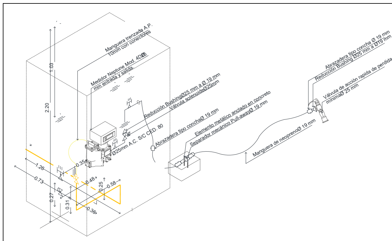
FIGURA III.1.3.7. DETALLE DE LA TOMA DE SUMINISTRO DE GAS LP DE LA ESTACIÓN | FUENTE: PLANO DEL PROYECTO MECÁNICO | ANEXO 3 EXPEDIENTE TÉCNICO DEL PROYECTO
