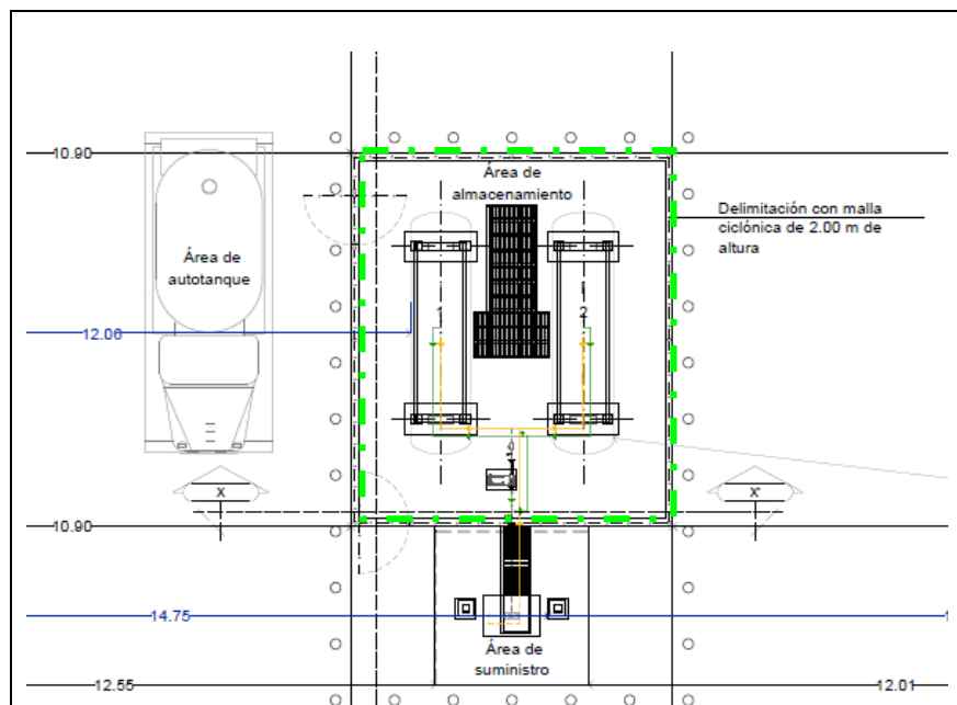
FIGURA III.1.3.3. ÁREA DE ALMACENAMIENTO DE LA ESTACIÓN | FUENTE: PLANOMÉTRICO Y PLANO DEL PROYECTO CIVIL | ANEXO 3 EXPEDIENTE TÉCNICO DEL PROYECTO
