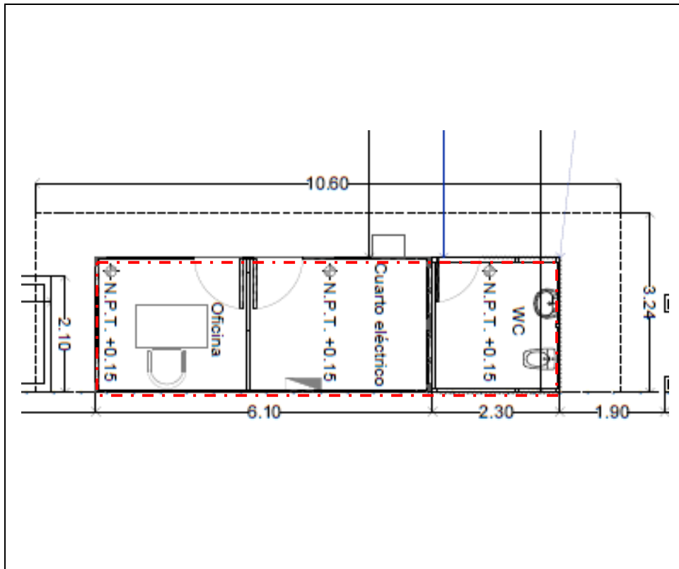
FIGURA III.1.3.2. EDIFICIO DE OFICINA Y SERVICIOS SANITARIOS DE LA ESTACIÓN | FUENTE: PLANO DEL PROYECTO PLANOMÉTRICO Y PLANO DEL PROYECTO CIVIL | ANEXO 3 EXPEDIENTE TÉCNICO DEL PROYECTO
