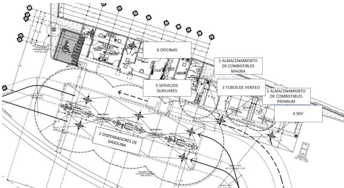
Figura 10. Diagrama de plano.
