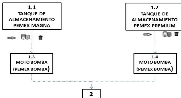
Figura 12. Diagrama de funcionamiento de almacenamiento de combustible.
