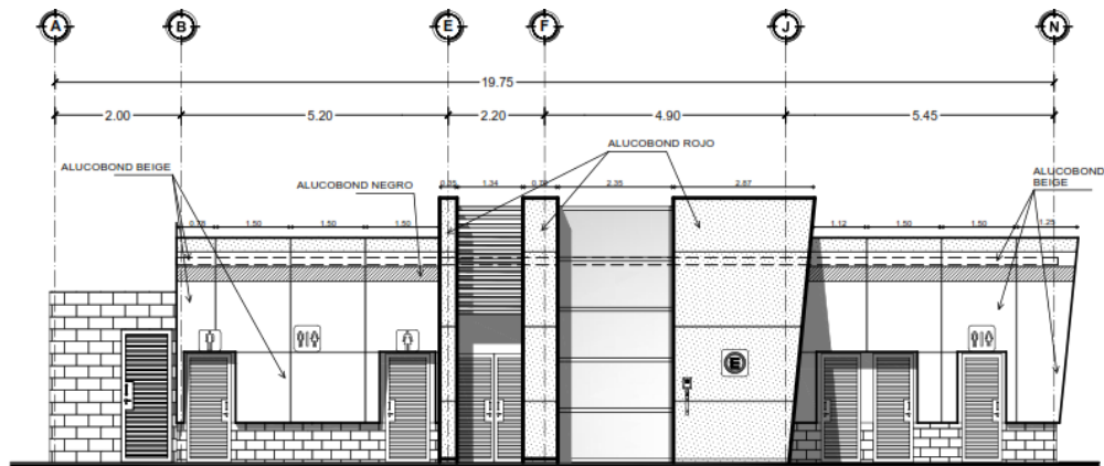
FACHADA PRINCIPAL EDIFICIO / SIN ESCALA
