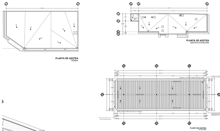
Plano 4. Plano de techumbre
