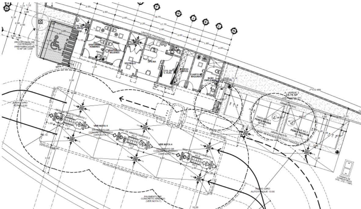
Plano 1. Plano de la estación.
