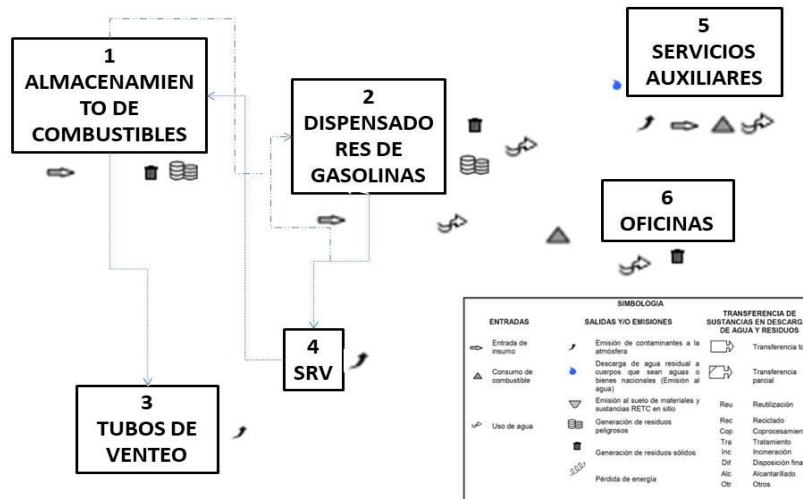
Figura 11. Diagrama de funcionamiento general de la Estación de Servicio.
