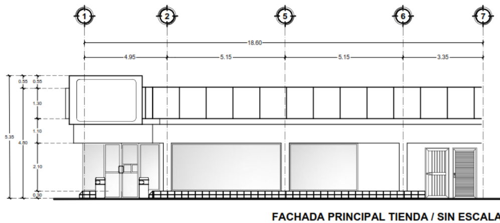
Plano 2. Plano de la fachada principal
