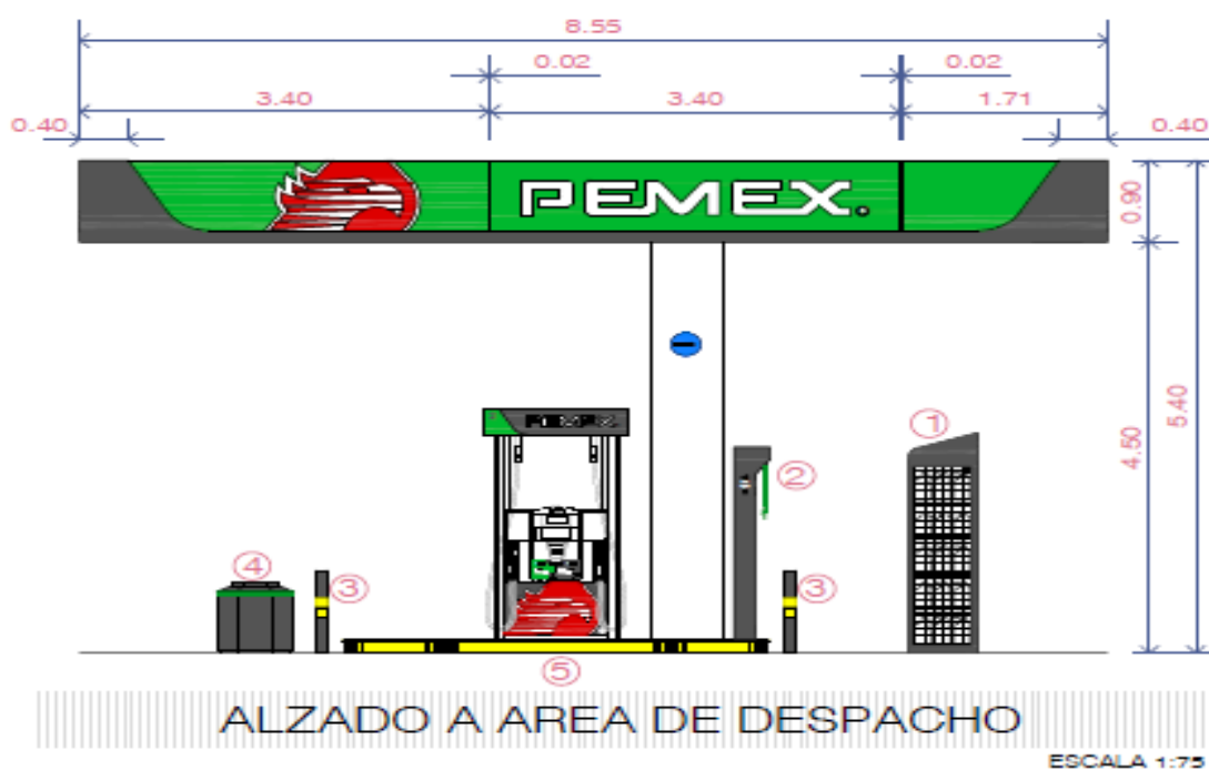
Alzado Frontal de Dispensario y Faldón.
