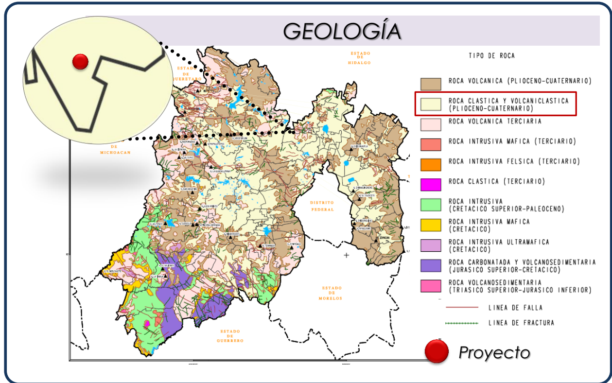
Figura 43 Geología
