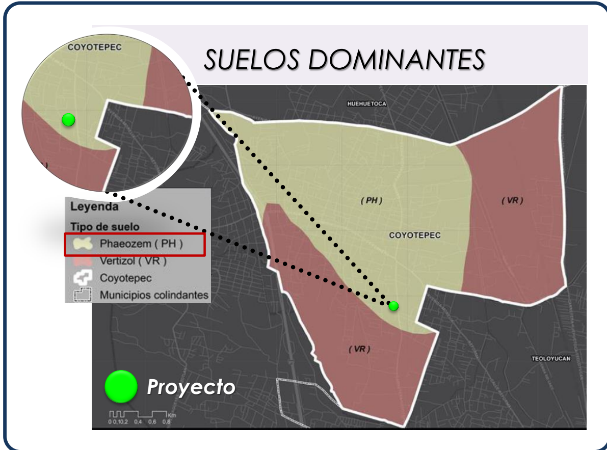
Figura 49 Suelos Dominantes
