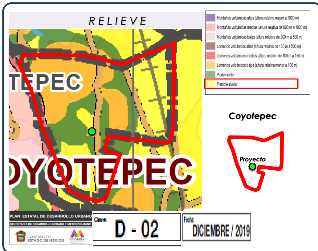
Figura 44 Relieve
