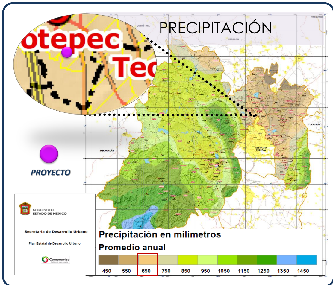
Figura 41 Precipitación promedio
