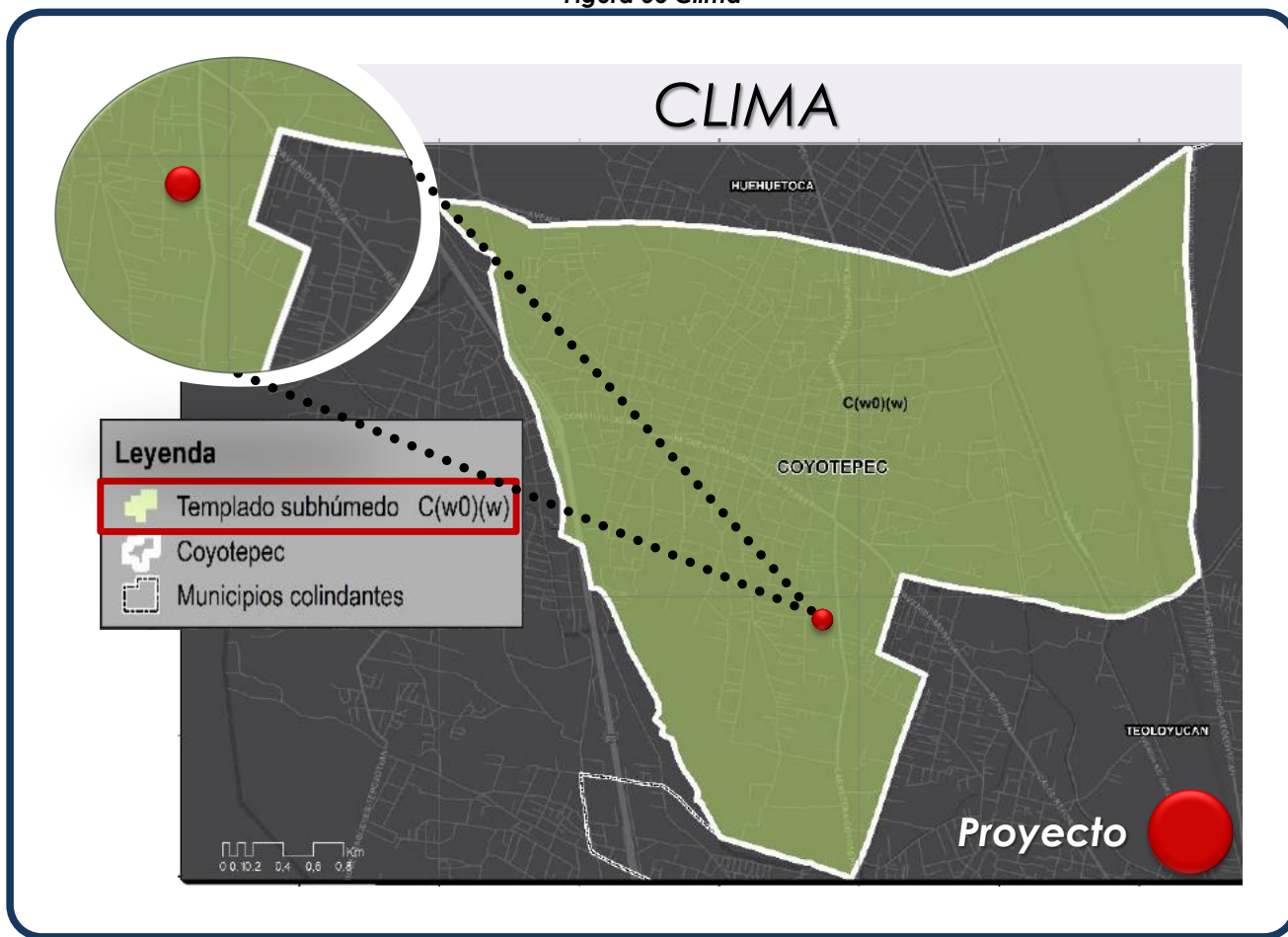
Figura 36 Clima
