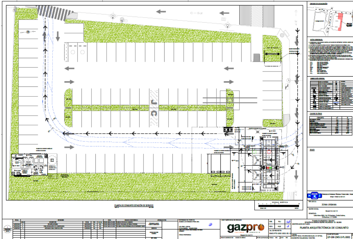
FIGURA 22. PLANO GENERAL DEL PROYECTO. ESPECIFICACIONES EN ANEXO 9
