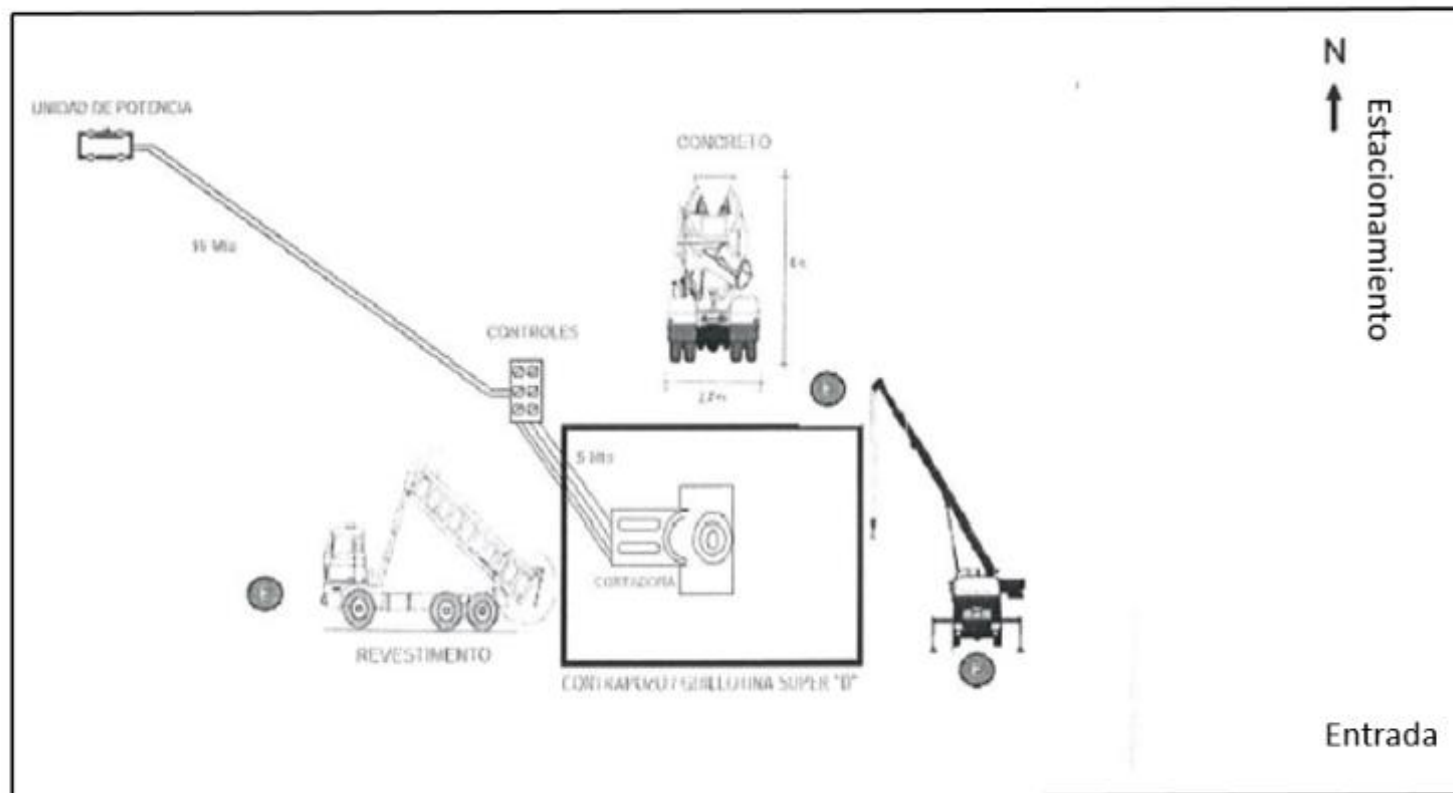
Figura I.1.5-3.- Distribución de la maquinaria y el equipo en el cuadro de maniobras para llevar a cabo el corte en frío para el tapón, colocación de manómetro, monumento y placa descriptiva.
