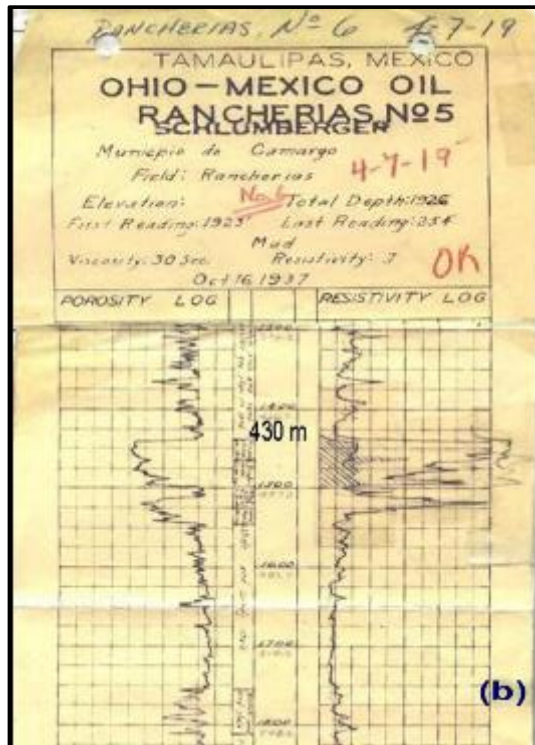
Figura III.1-3.- Registros de pozo del sondeo Rancherías 5.
