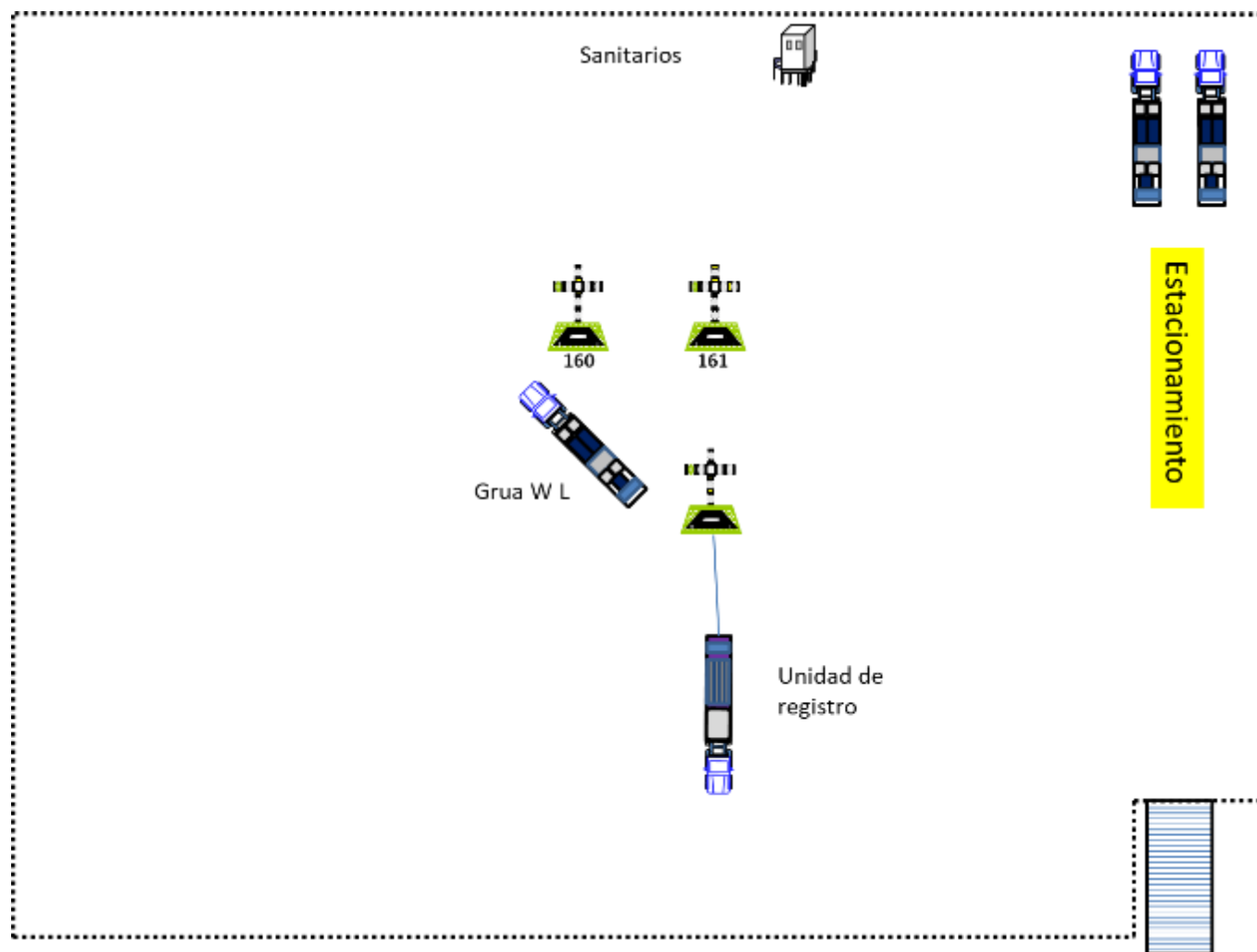
Figura I.1.5-2.- Distribución de la maquinaria y el equipo en el cuadro de maniobras para llevar a cabo los disparos de los pozos para taponamiento.
