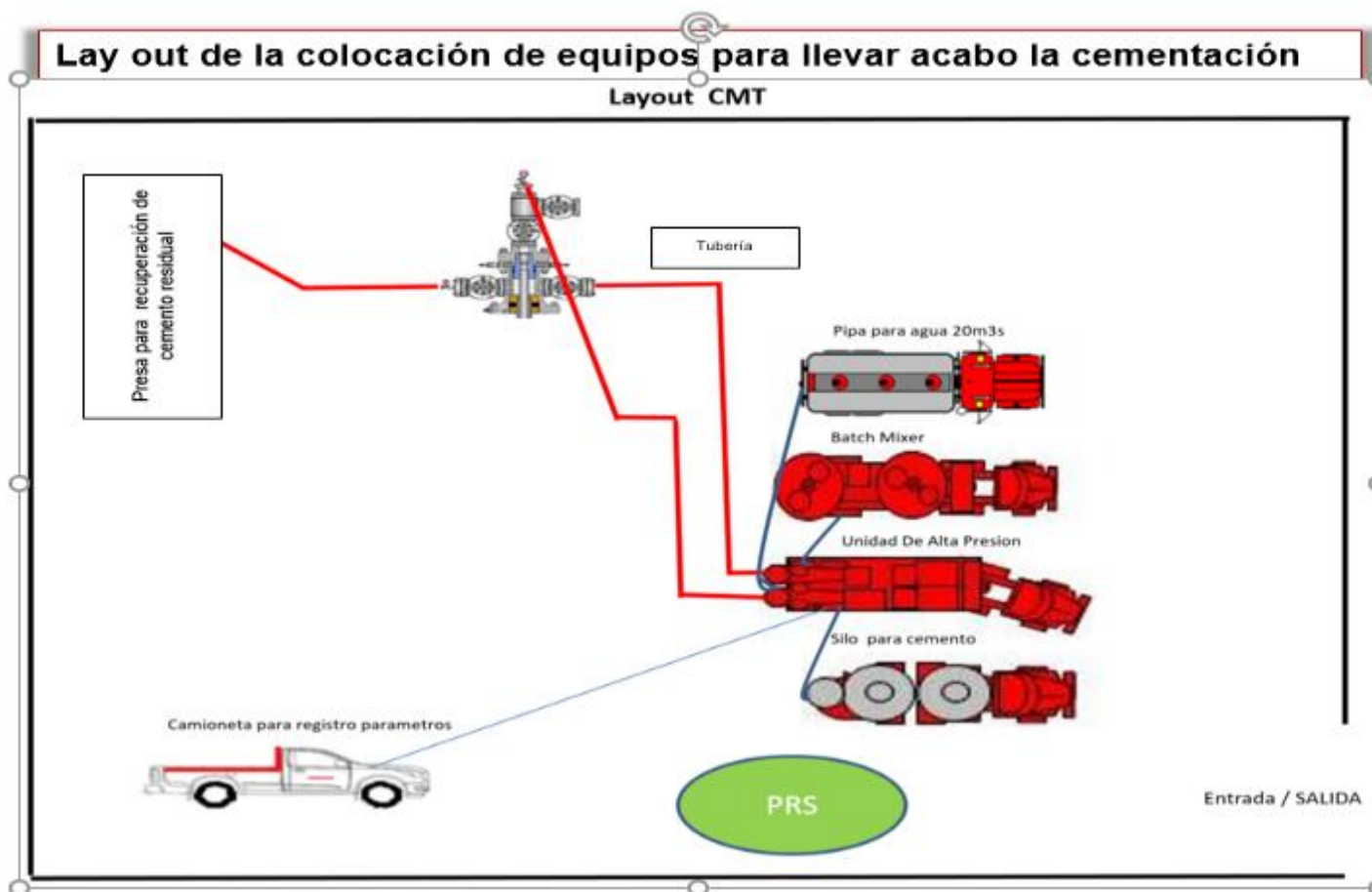
Figura I.1.5-1.- Distribución de la maquinaria y el equipo en el cuadro de maniobras para llevar acabo la cementación de los pozos para taponamiento.
