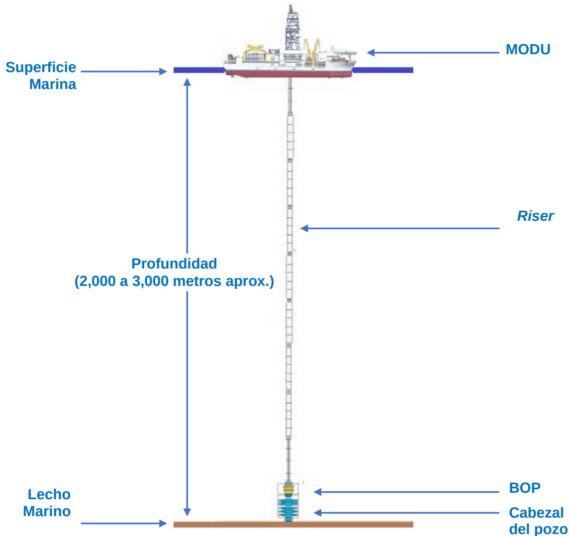
Figura 2-4. Diagrama de un buque de perforación típico con riser y BOP instalados.
