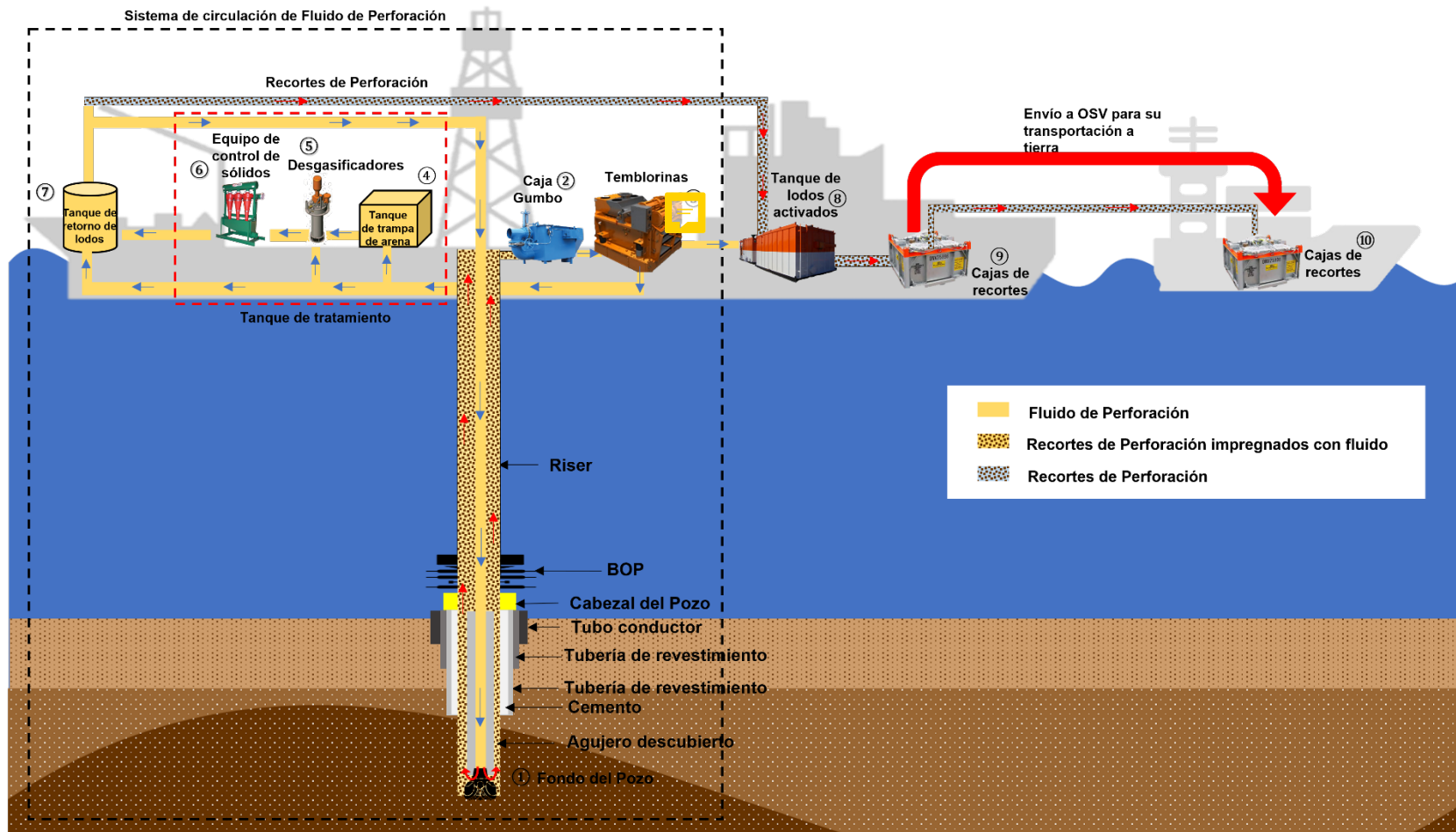
Figura 2-8. Diagrama del proceso de recirculación típico de los recortes de perforación y su transporte.
