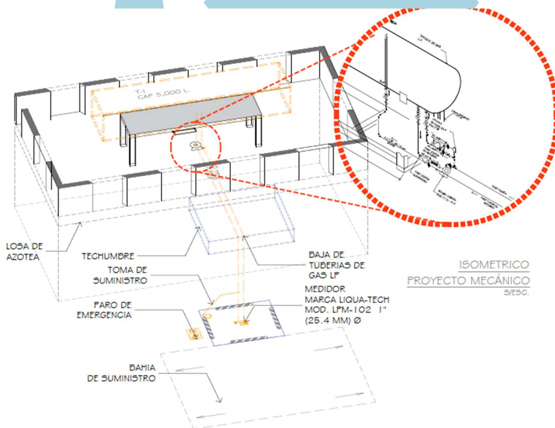
Imagen 8. Isométrico de la Estación de Carburación para gas L.P.
