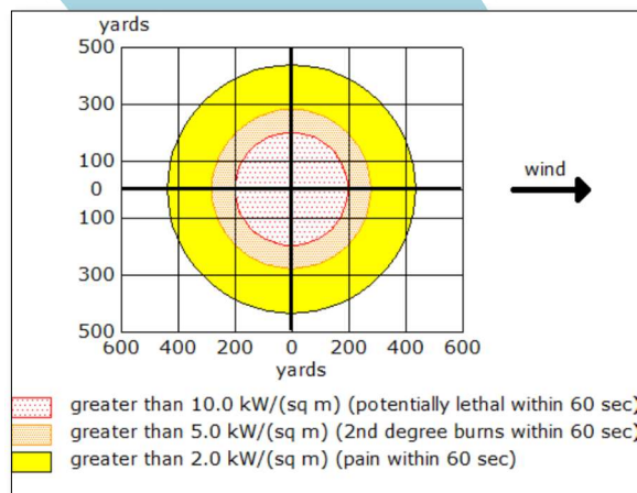
Imagen 12. Escenario catastrófico Aloha.
