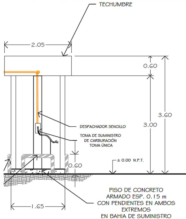
Imagen 10. Vista Longitudinal de la Toma de Suministro.
