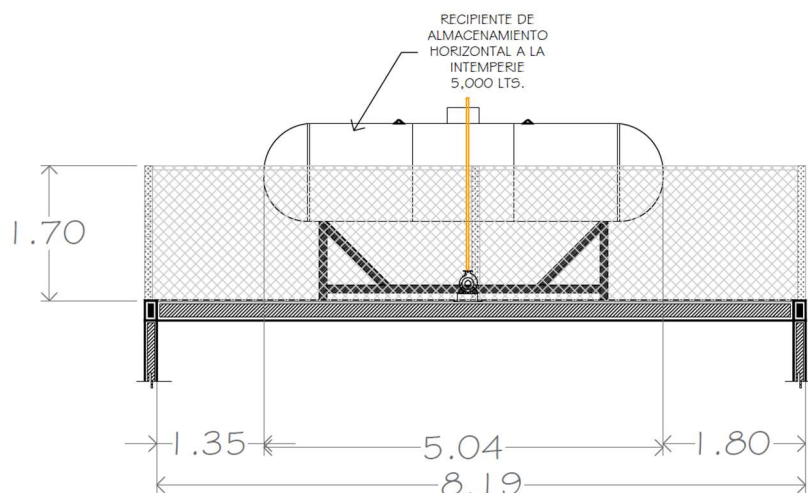
Imagen 9. Vista Longitudinal del Tanque de Almacenamiento.
