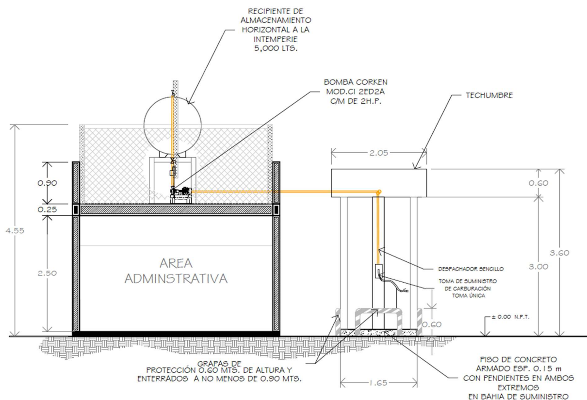
Imagen 6. Vista Frontal de la Estación de Gas L.P. para Carburación.
