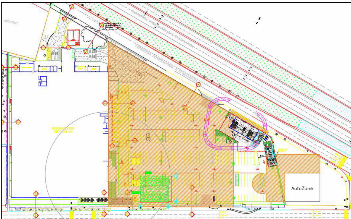
FIGURA 5. PLANO GENERAL DEL PROYECTO.
