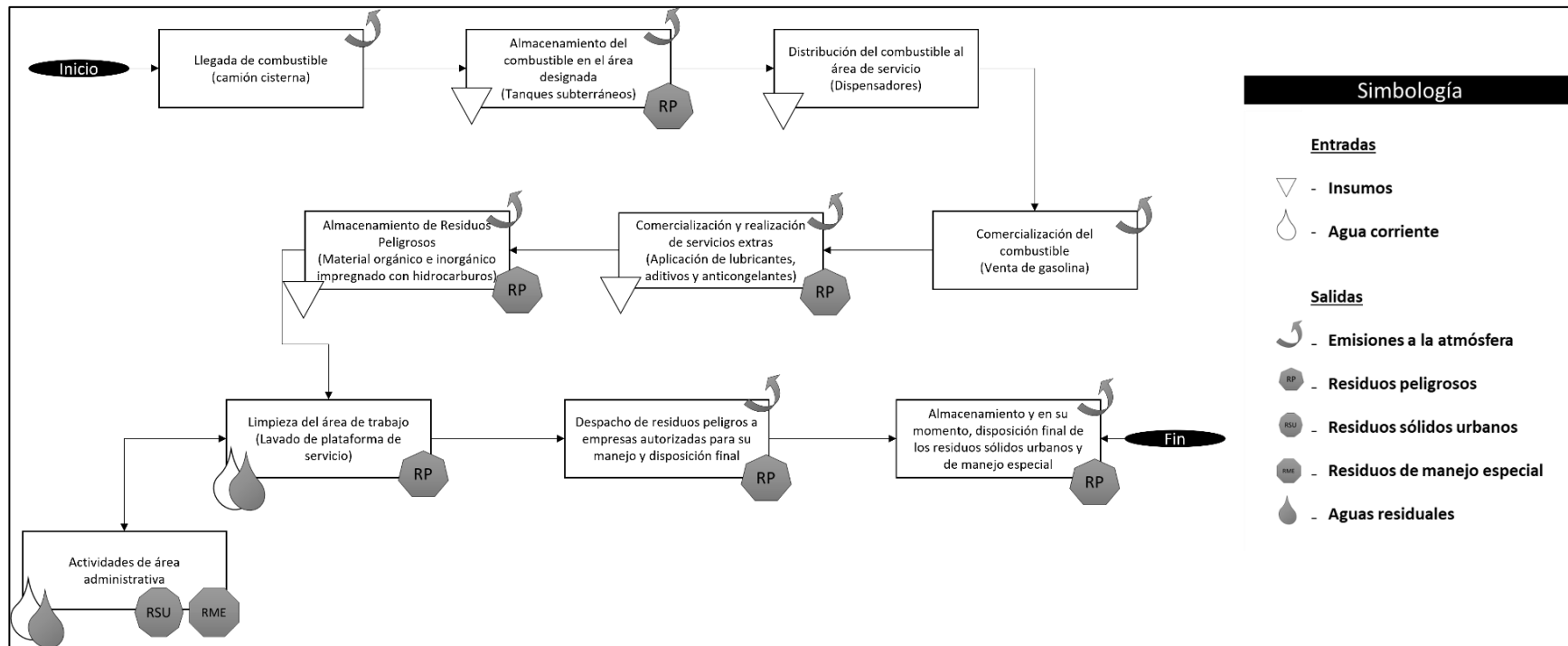
FIGURA 7. DIAGRAMA DE PROCESOS PARA LA COMERCIALIZACIÓN DE HIDROCARBUROS E IDENTIFICACIÓN DE SUS EMISIONES, DESCARGAS Y GENERACIÓN DE RESIDUOS
