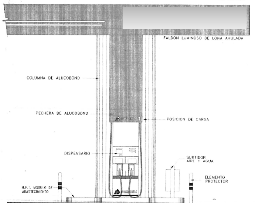
Alzado Frontal de Dispensario y Faldón.
