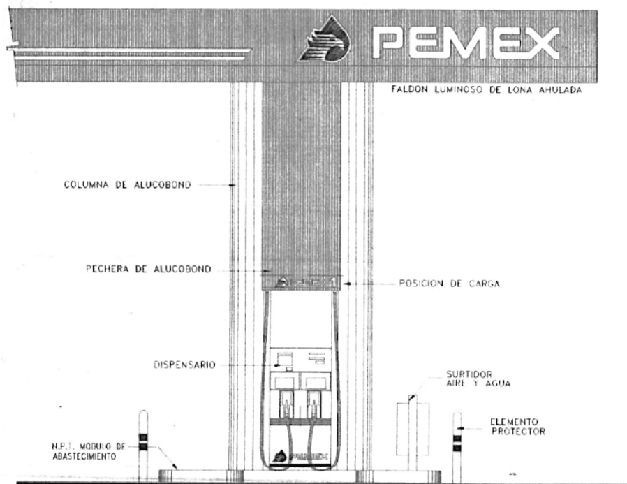
Imagen 8. Alzado Frontal de Dispensario y Faldón.
