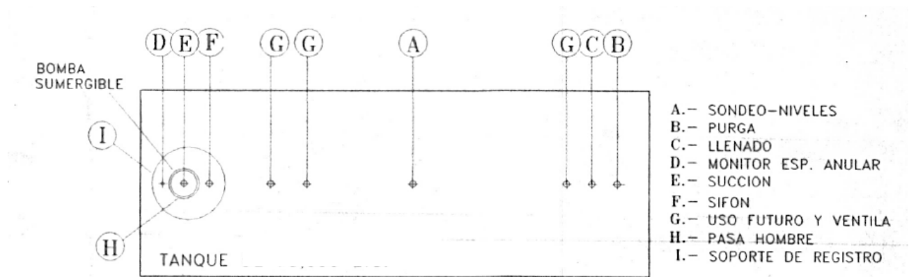
Imagen 9. Accesorios tanques de almacenamiento.
