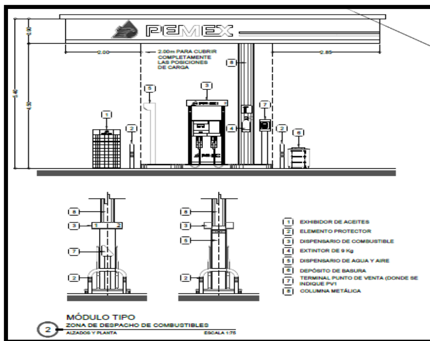
Imagen 12. Diagrama Tipo del Módulo de Abastecimiento.
