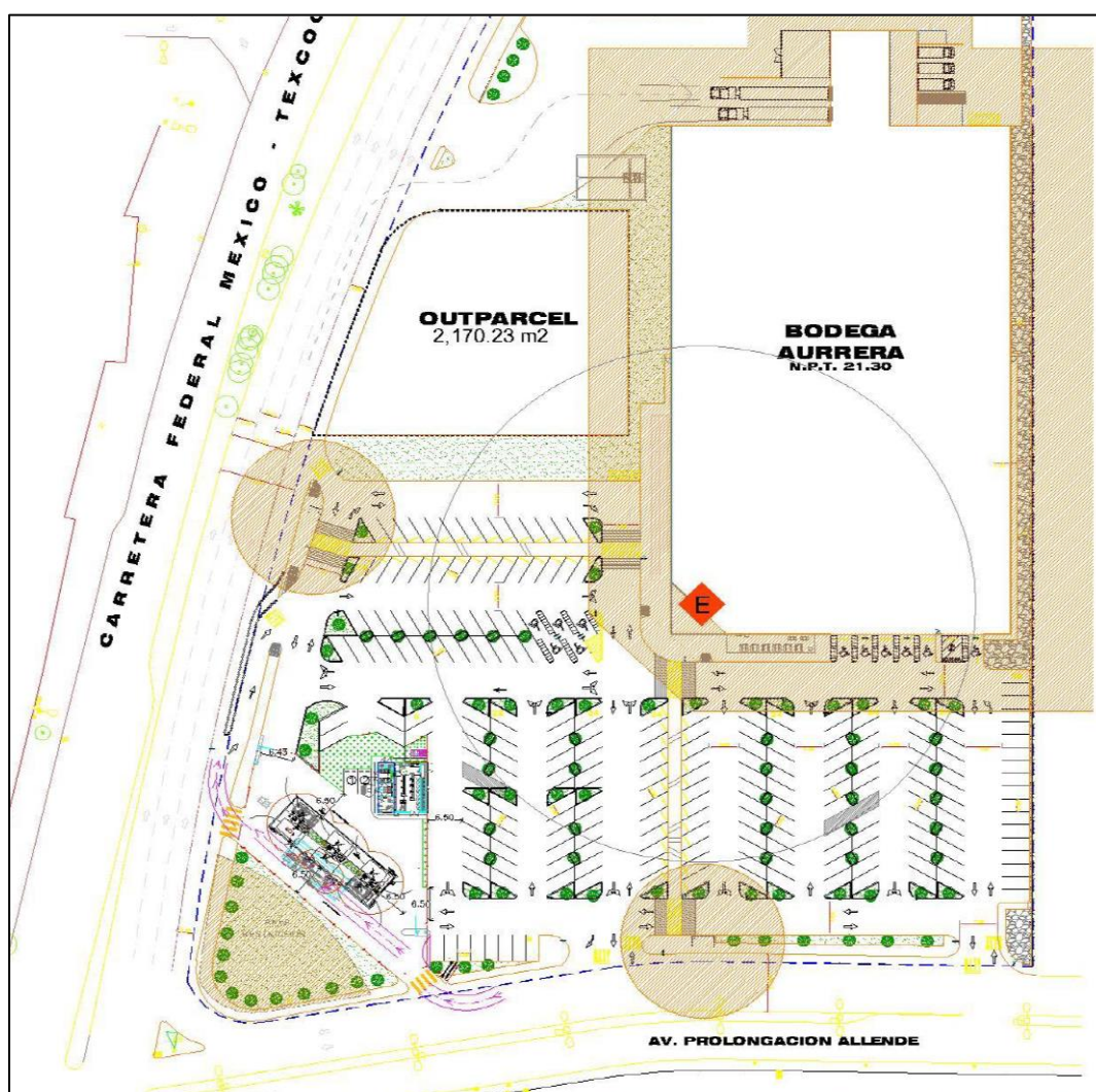
FIGURA 4. HUELLA DE LA ESTACIÓN DE SERVICIO EN EL ESPACIO DE LA TIENDA
