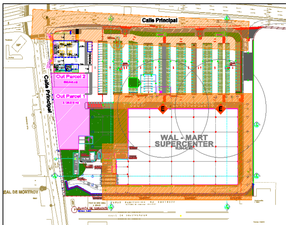
FIGURA 4. HUELLA DE LA ESTACIÓN DE SERVICIO EN EL ESPACIO DE LA TIENDA
