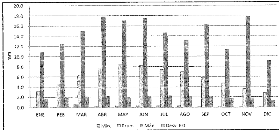
FIGURA 16. VALORES HISTÓRICOS DE EVAPORACIÓN POR MESES EN EL PERIODO 1975-2013 EN LERDO. FUENTE (SMN, 2020)
